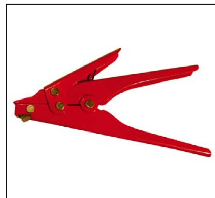
Outils de serrage et de coupe pour collier en Nylon 3.6 - 13.0mm
