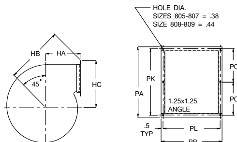
OPTIONAL OUTLET FLANGE
