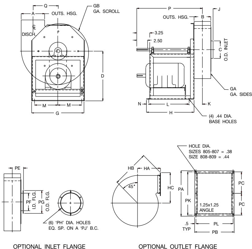
OPTIONAL INLET FLANGE
