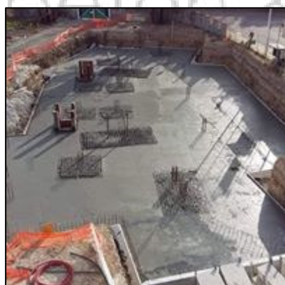
Foto_Nelle immagini getto per platea in Rck40 eseguito a Cagliari per la realizzazione di fondazione impermeabilizzata, getto in continuo di mc 350
