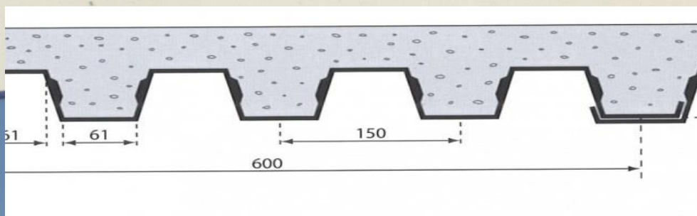
Figura 2 LAMIERE ZINCATE GRECATE 600-55 COLLABORANTE, PER SOLAI
