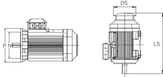
Flange-mounted motor IM 3001, IM B5
