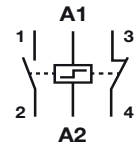
E290-16-11/230 Relè passo-passo Modulo principale
