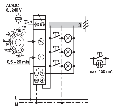
E 232E-8/230 Multi 10 Configurazione a 3 fili
