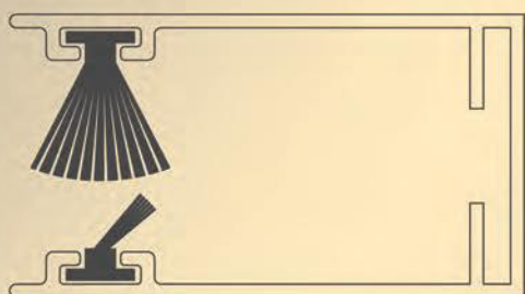
Sezione guida antivento
