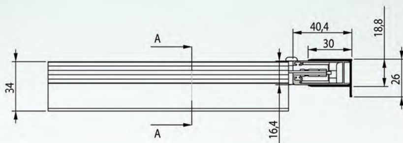
SEZIONE B-B
