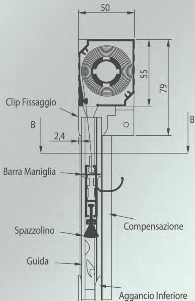
SEZIONE A-A
