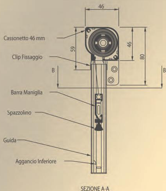
SEZIONE A-A
