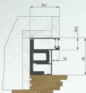
Guida senza rivestimento in legno
