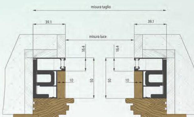
Guida con rivestimento in legno
