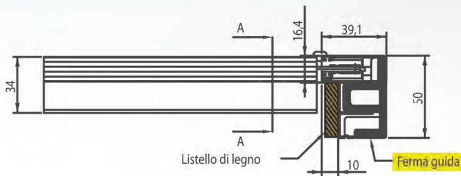
SEZIONE B-B
