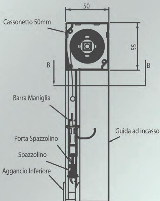
SEZIONE A-A
