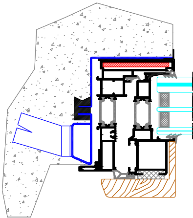
ALLUMINIO IN BATTUTA ALLUMINIUM CLOSES FERME EN ALUMINIUM IKONA / IKONA WOOD
