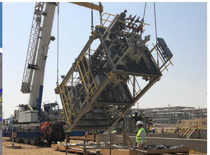
Piattaforme e grossi insiemi SKID e PIPING
