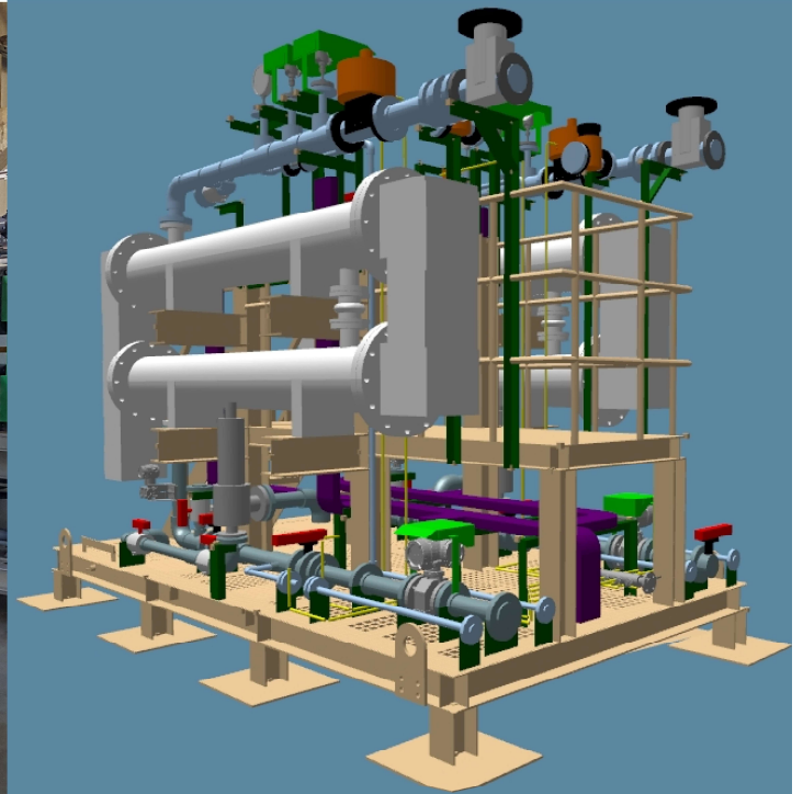
Singoli SKID di piccola e media dimensione
