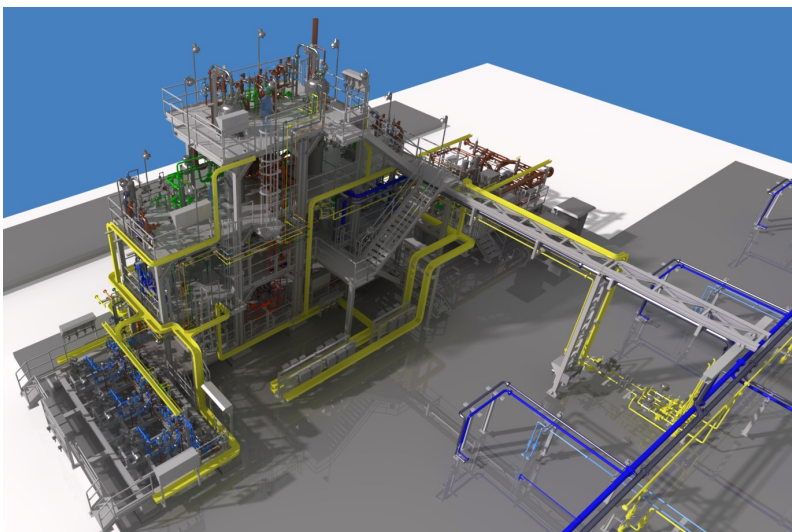
Piattaforme e grossi insiemi SKID e PIPING
