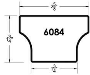
R6084
