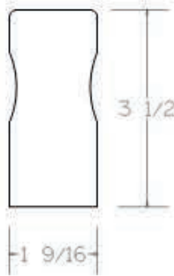
R6048
