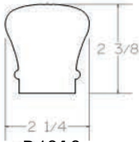
R6010
