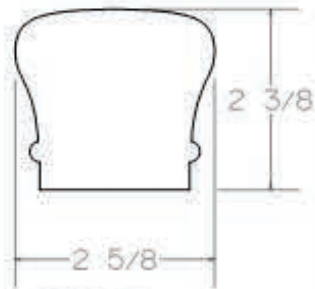
R6210
