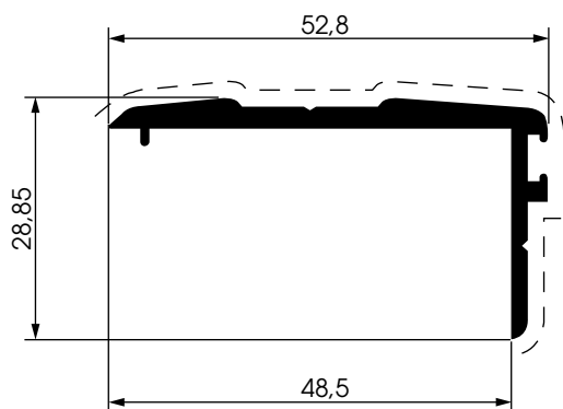
9845 peso: Kg./mt. 0.548 sup. in vista: mm. 171
