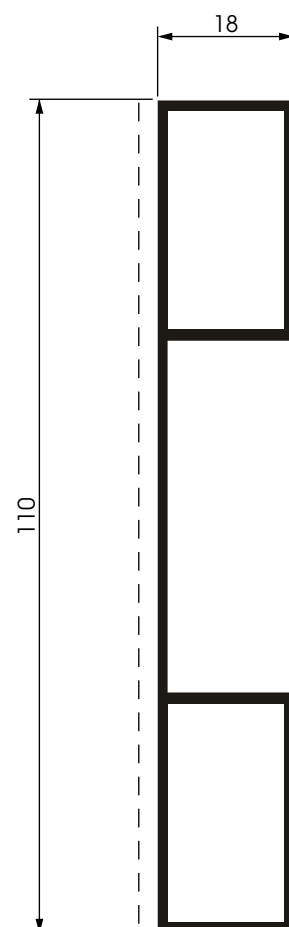
9848 peso: Kg./mt. 1.015 sup. in vista: mm. 110
