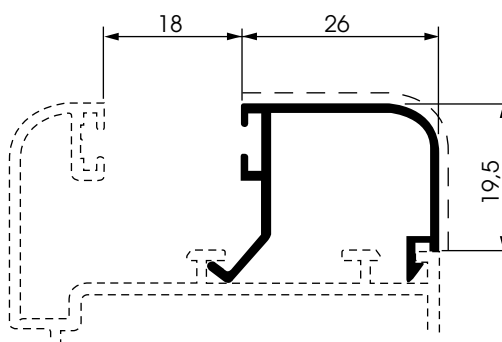
9627/18T peso: Kg./mt. 0.272 sup. in vista: mm. 44
