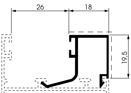
9624/26 peso: Kg./mt. 0.270 sup. in vista: mm. 37
