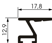
9847 peso: Kg./mt. 0.178 sup. in vista: mm. 0
