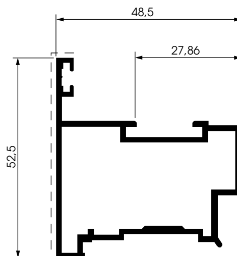
9816 peso: Kg./mt. 0.859 sup. in vista: mm. 74
