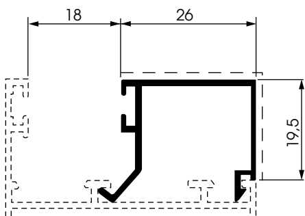
9622/18 peso: Kg./mt. 0.275 sup. in vista: mm. 45
