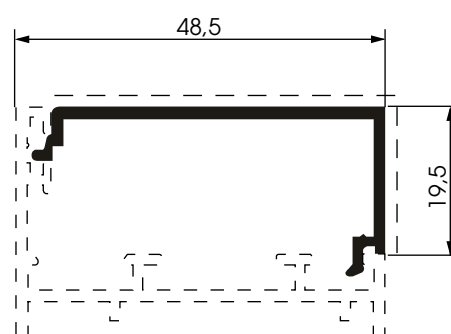
9846 peso: Kg./mt. 0.302 sup. in vista: mm. 68
