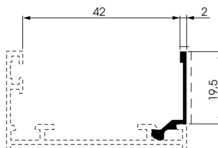
9626/42 peso: Kg./mt. 0.110 sup. in vista: mm. 21
