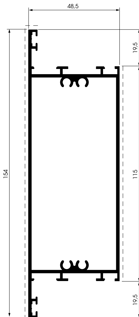
9818 peso: Kg./mt. 2.009 sup. in vista: mm. 269
