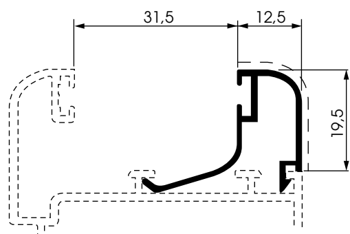
9629/31,5T peso: Kg./mt. 0.255 sup. in vista: mm. 30
