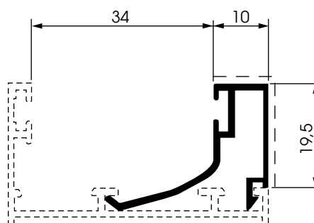
9625/34 peso: Kg./mt. 0.255 sup. in vista: mm. 30
