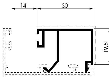
9829/14 peso: Kg./mt. 0.330 sup. in vista: mm. 50
