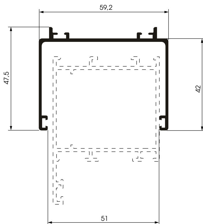
9834 peso: Kg./mt. 0.800 sup. in vista: mm. 94
