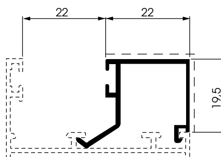
9623/22 peso: Kg./mt. 0.276 sup. in vista: mm. 41
