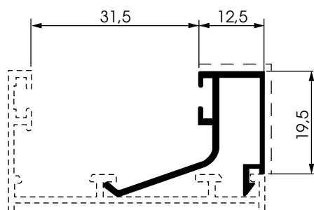
9650/31,5 peso: Kg./mt. 0.267 sup. in vista: mm. 32
