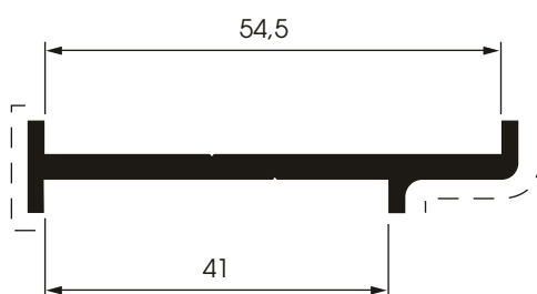
9693 peso: Kg./mt. 0.560 sup. in vista: mm. 39,5
