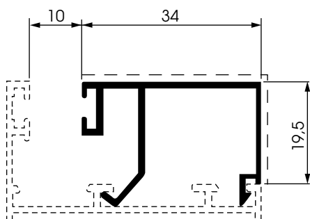
9820/10 peso: Kg./mt. 0.340 sup. in vista: mm. 53
