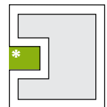
Con tacca * Dimensioni minime della tacca (zona verde) 5 x 7 cm oppure 7 x 5 cm
