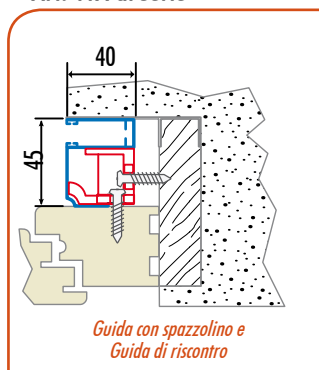
Art. 11A di serie
