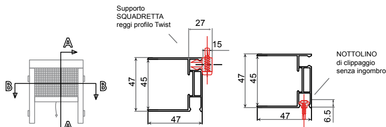
Configurazione "Invertita" barramaniglia Alta
