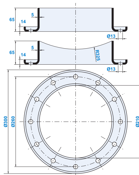
Bride Ø300 à 12 trous
