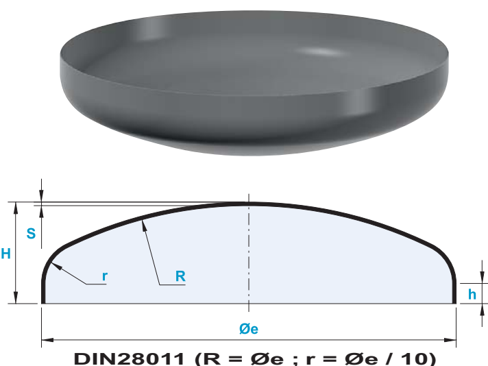
Tipo di bordatura eseguibile
