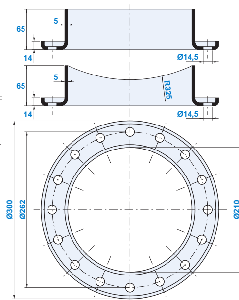
Flangia 16 fori + Taglio al plasma R325 Bride 16 trous + Découpe au plasma R325
