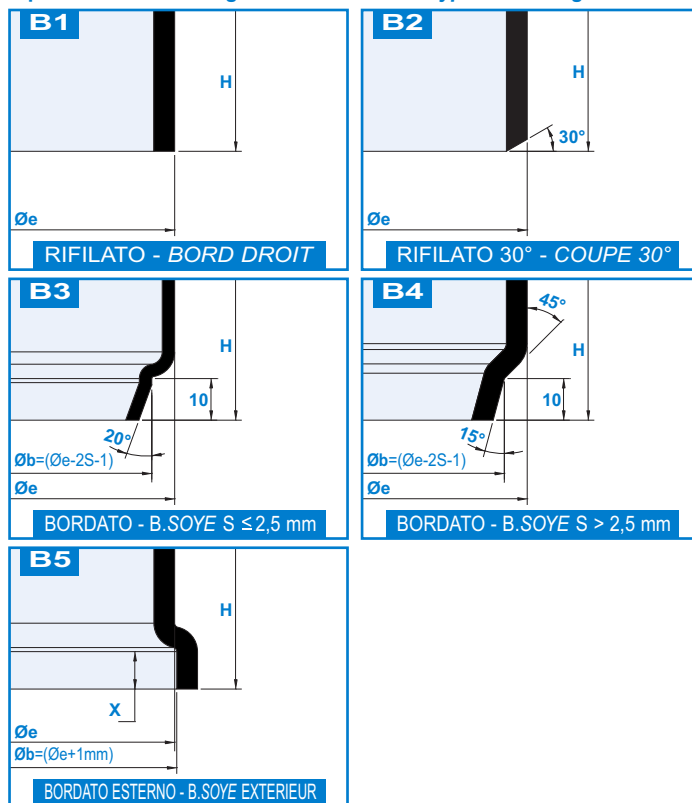
Tipo di bordatura eseguibile
