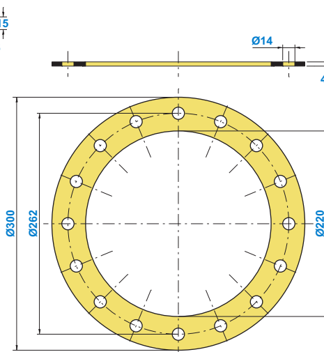
Guarnizione Joint
