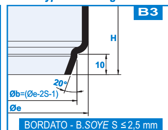
Type de bordage réalisable
