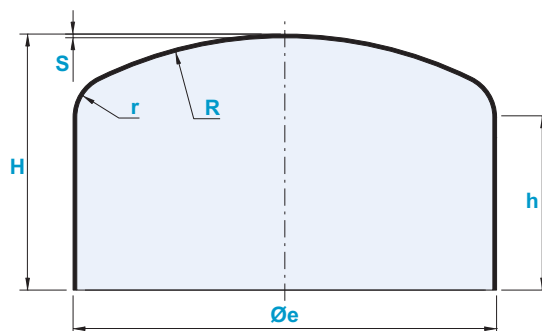
Tipo di bordatura eseguibile
