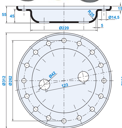
Coperchio 16 fori con n°2 fori Ø42 senza fori Ø42 Couvercle 16 trous avec n°2 trous Ø42 sans trous Ø42
