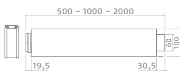
Tronchetto ispezione
