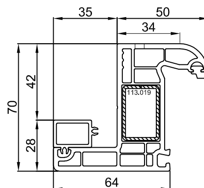
TELAIO 101.219.34
