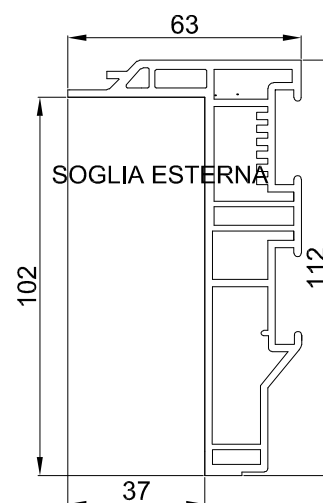
PROFILO ISO/ECOALAF37S102 ISOLTEK/ECOTEK CON ZANZARIERA UTILIZZO NASTRO 3E
