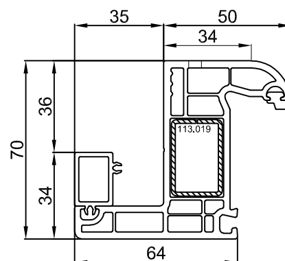
TELAIO 101.219.34
