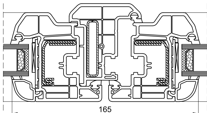
NODO BATTUTA CENTRALE (STANDARD) CON PROFILO DI SCAMBIO BATTUTA 102.236
