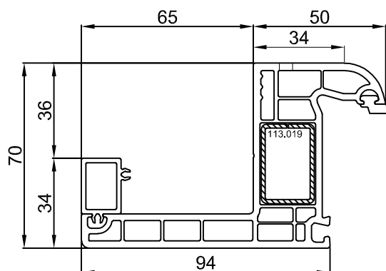
TELAIO 101.229.34
