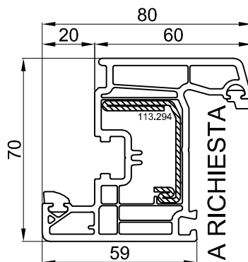
ANTA MAG. AP. EST. 103.242
