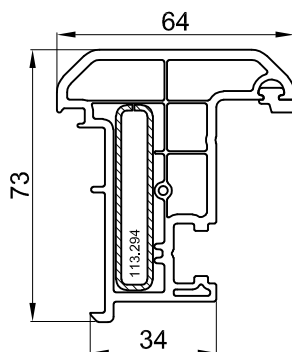
SC.BATTUTA 102.236
