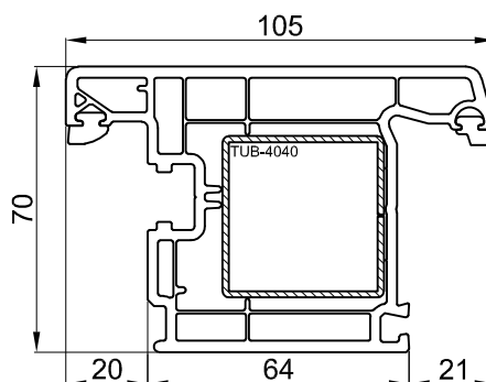
PIANTONE-TRAVERSO 102.238
