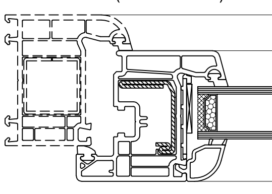
ANTA 103.232 (A RICHIESTA)
