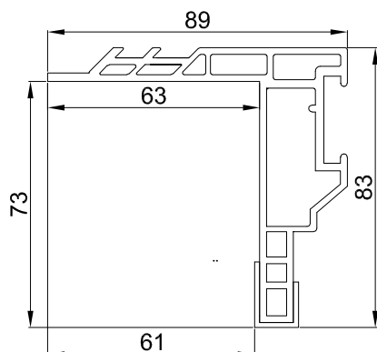
PROFILO ISO/ECOCPF63S73 ISOLTEK/ECOTEK SENZA ZANZARIERA UTILIZZO NASTRI BG1+3EUA
