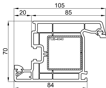
ANTA MAGGIORATA 103.241
