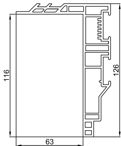
FALSO TELAIO
