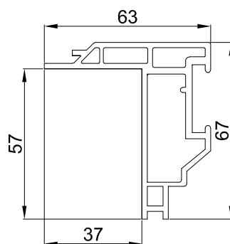
PROFILO ISO/ECOALAF37S57 ISOLTEK/ECOTEK SENZA ZANZARIERA UTILIZZO NASTRO 3E
