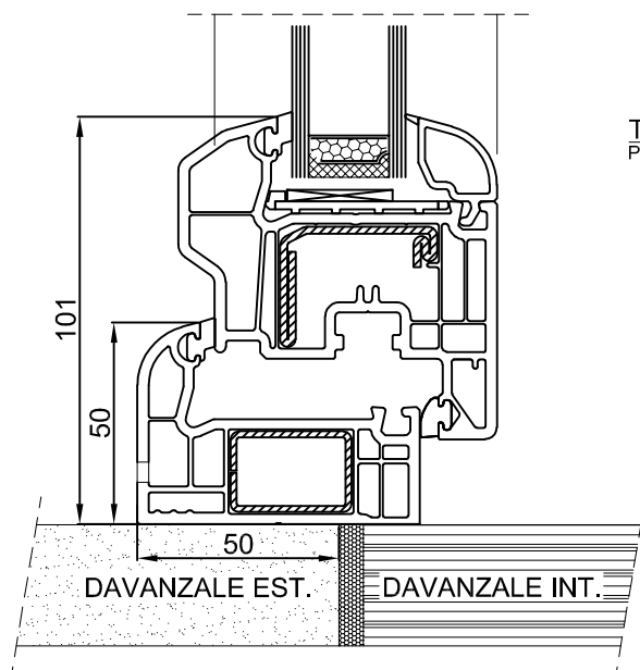
ZOCCOLO OPTIONAL PROFILO 105.130
