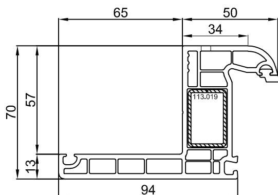
TELAIO 101.229
