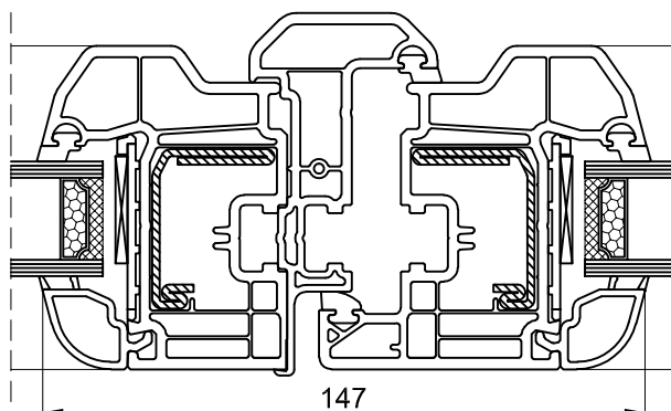
NODO BATTUTA CENTRALE (A RICHIESTA) CON PROFILO DI SCAMBIO BATTUTA 102.219
