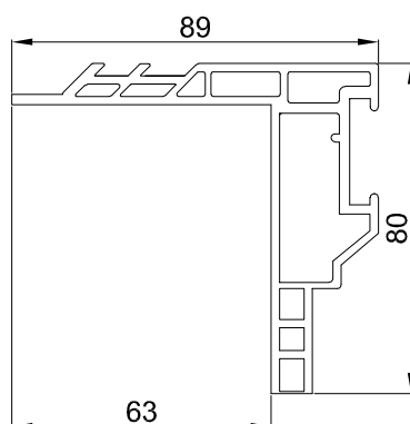
PROFILO ISO/ECOCPF63S70 ISOLTEK/ECOTEK SENZA ZANZARIERA UTILIZZO NASTRO 3E
