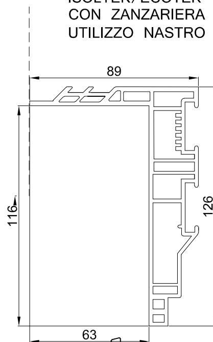
PROFILO ISO/ECOCPF63S116 ISOLTEK/ECOTEK CON ZANZARIERA UTILIZZO NASTRO 3E
