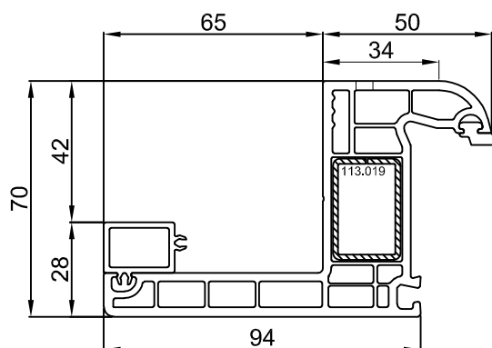
TELAIO 101.229.34
