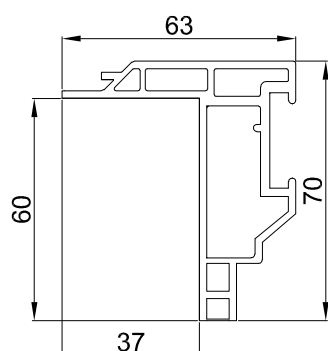
PROFILO ISO/ECOALAF37S60 ISOLTEK/ECOTEK SENZA ZANZARIERA UTILIZZO NASTRI BG1+3EUA
