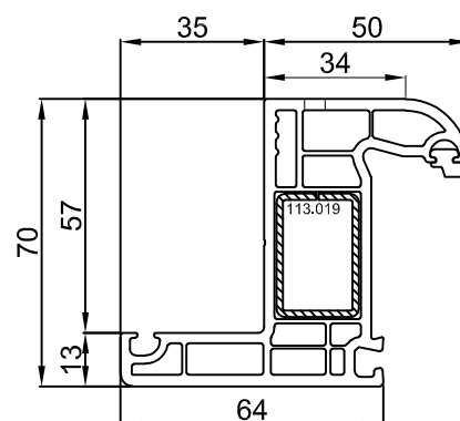
TELAIO 101.219.28
