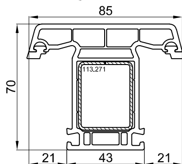
PIANTONE-TRAVERSO 102.218
