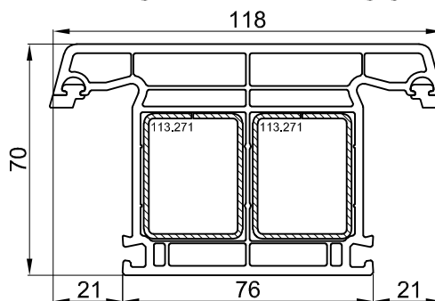
PIANTONE-TRAVERSO 102.238
