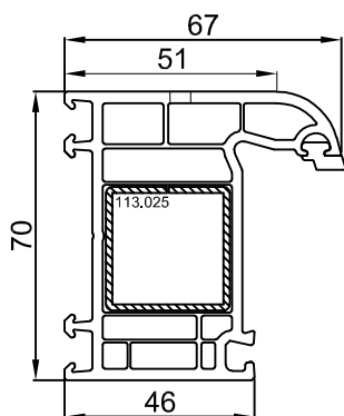
TELAIO 101.233
