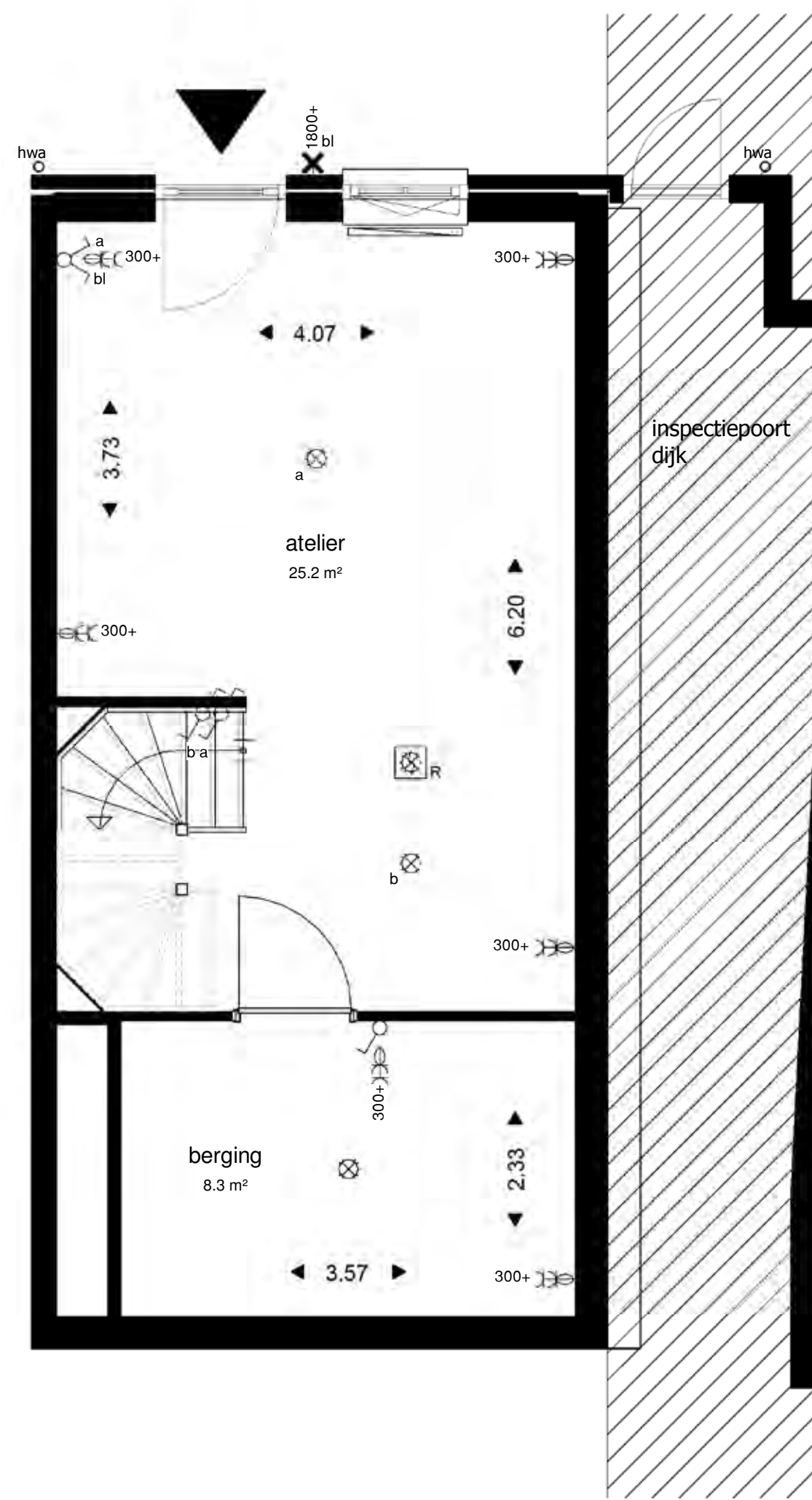
kelder
