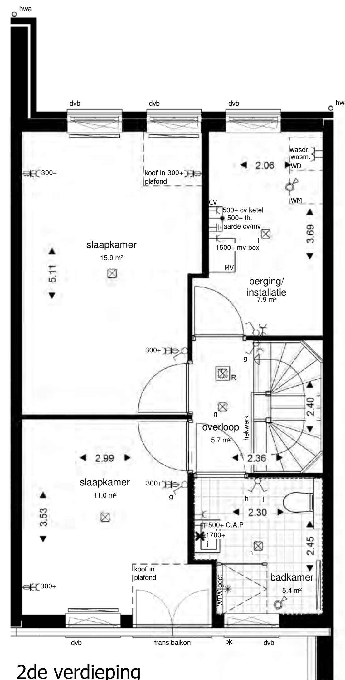
2de verdieping
