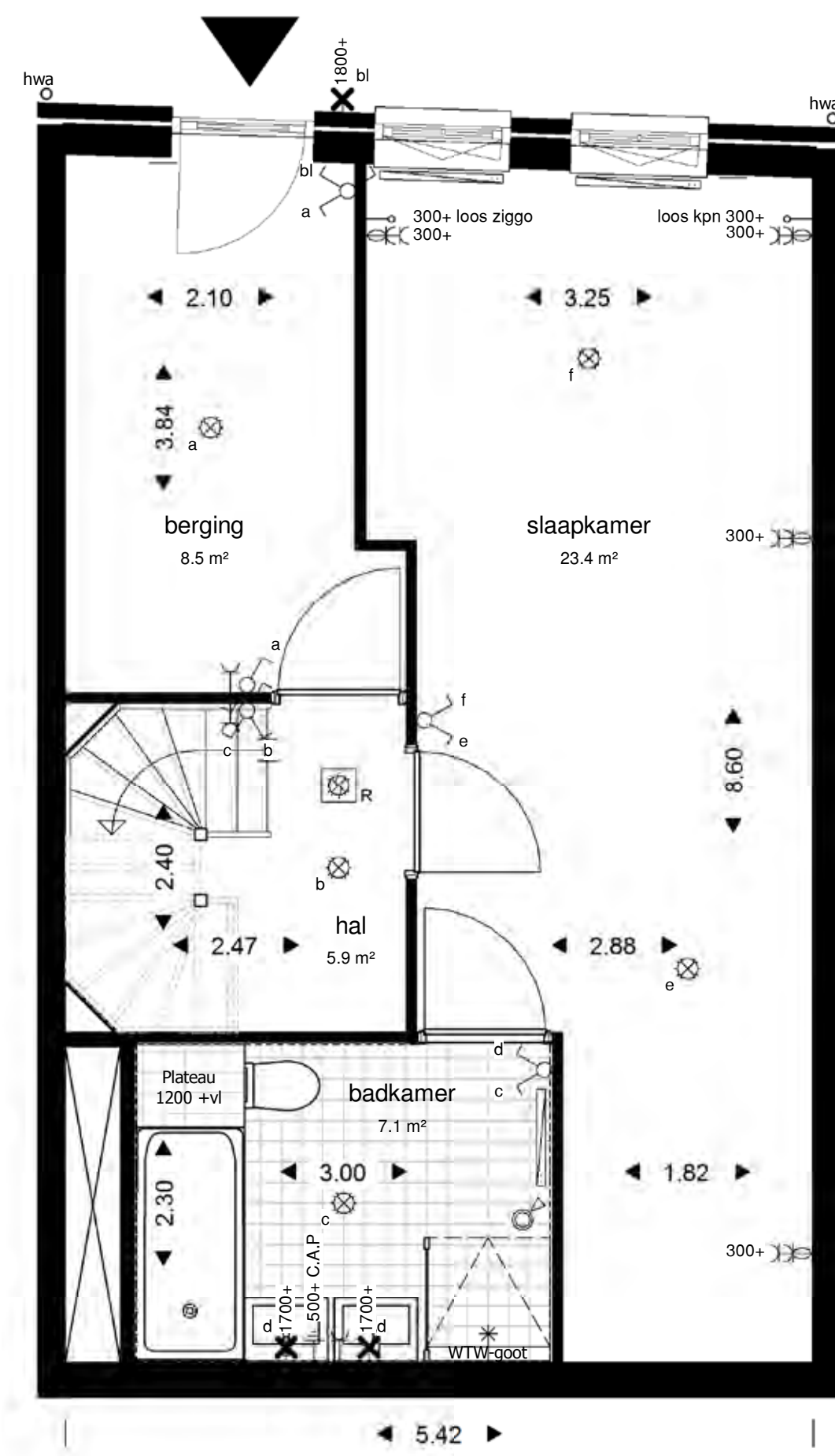
kelder
