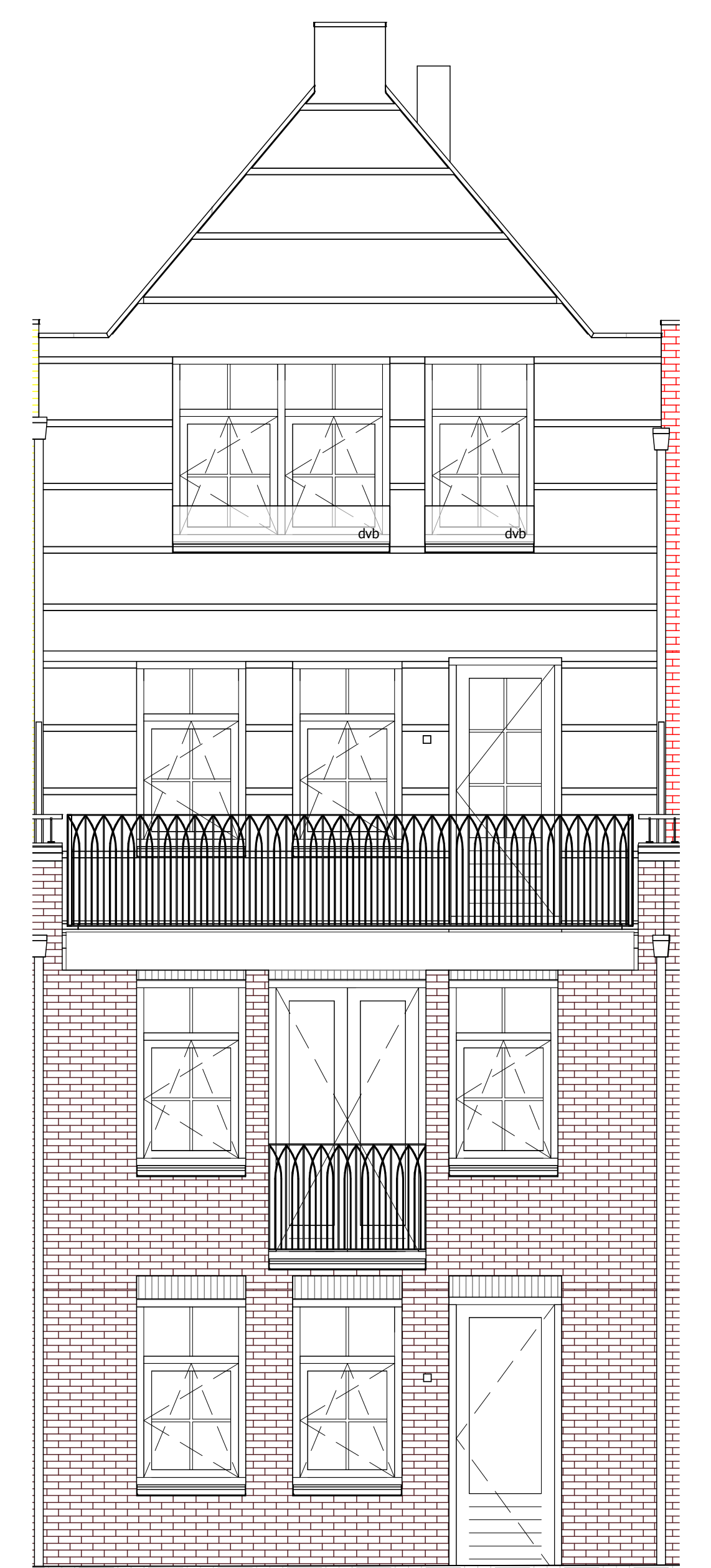
achtergevel
