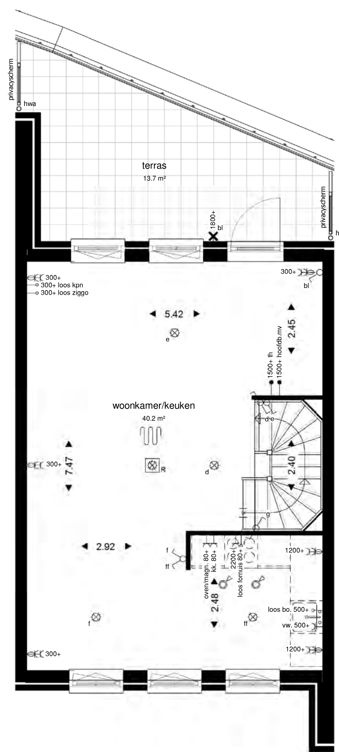
1ste verdieping
