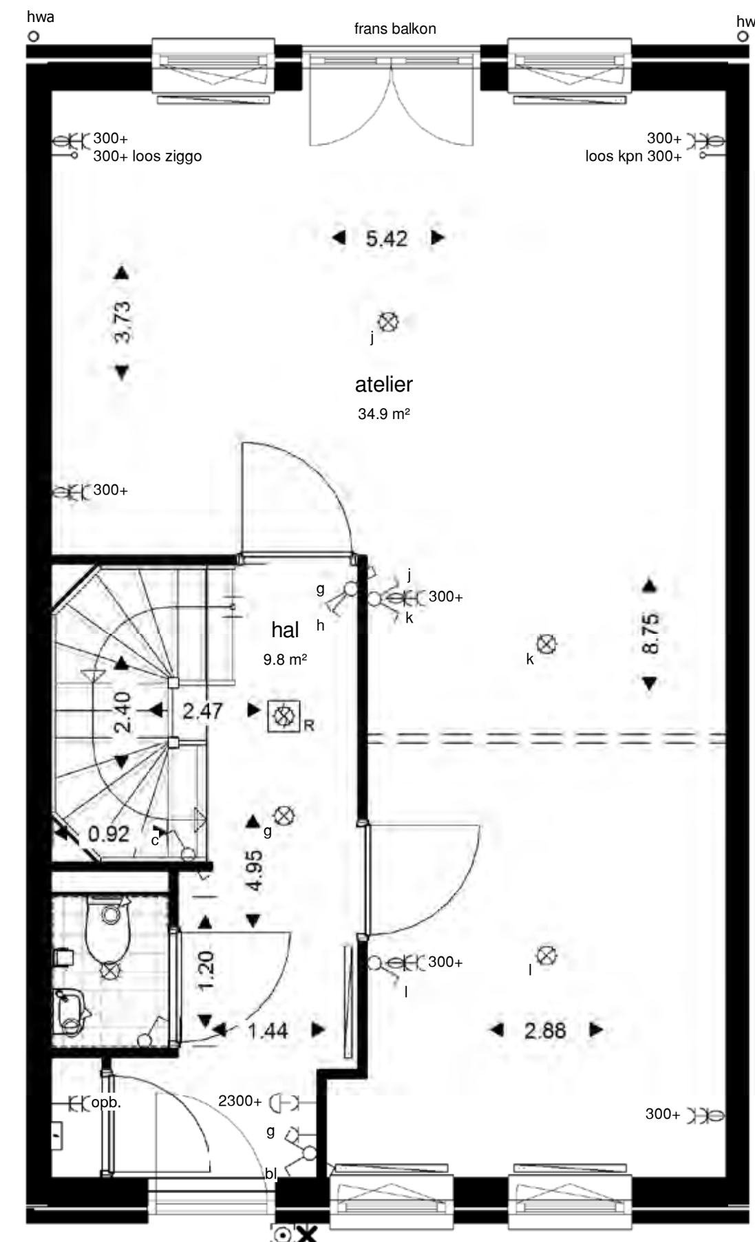
begane grond
