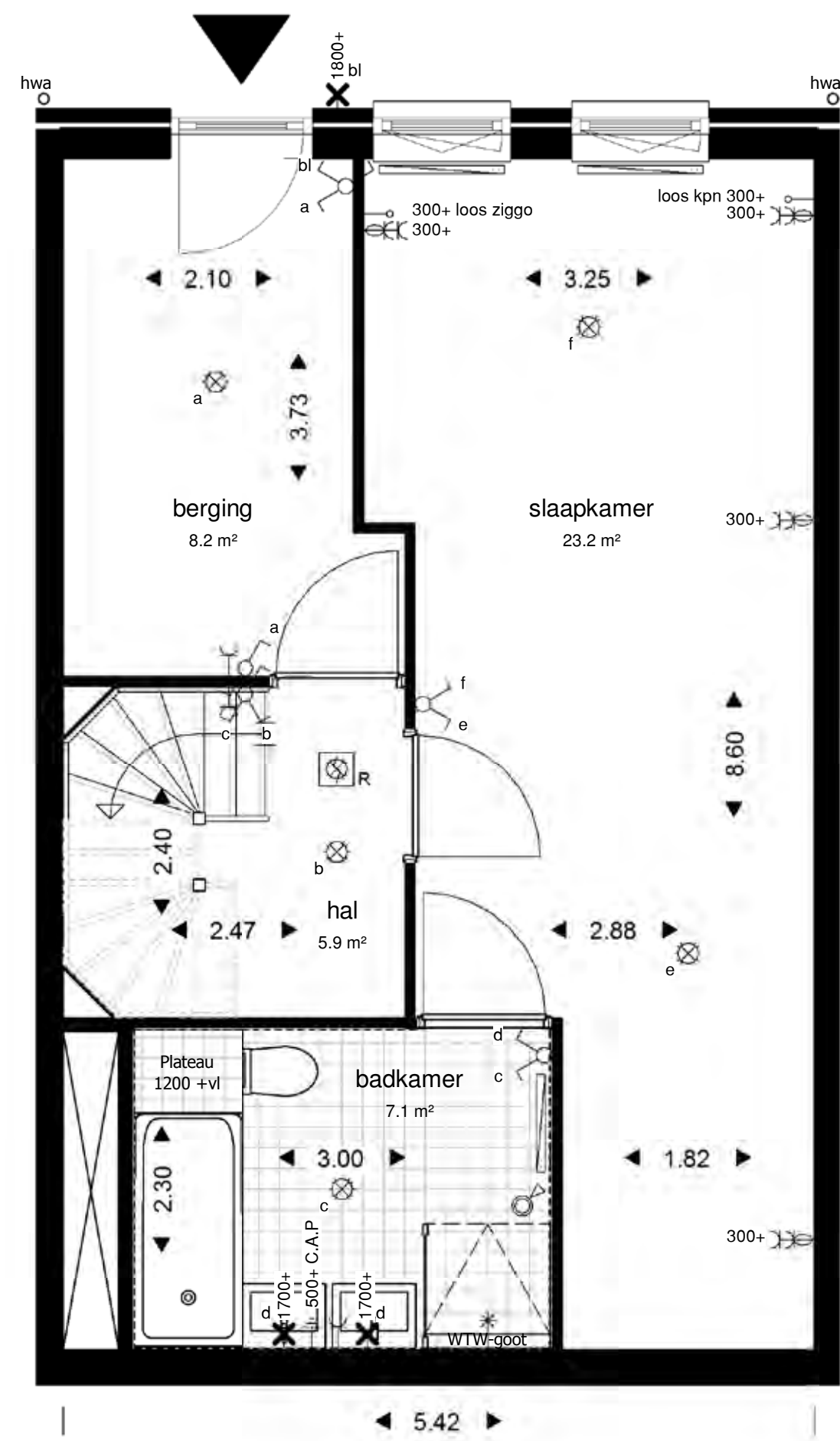
kelder
