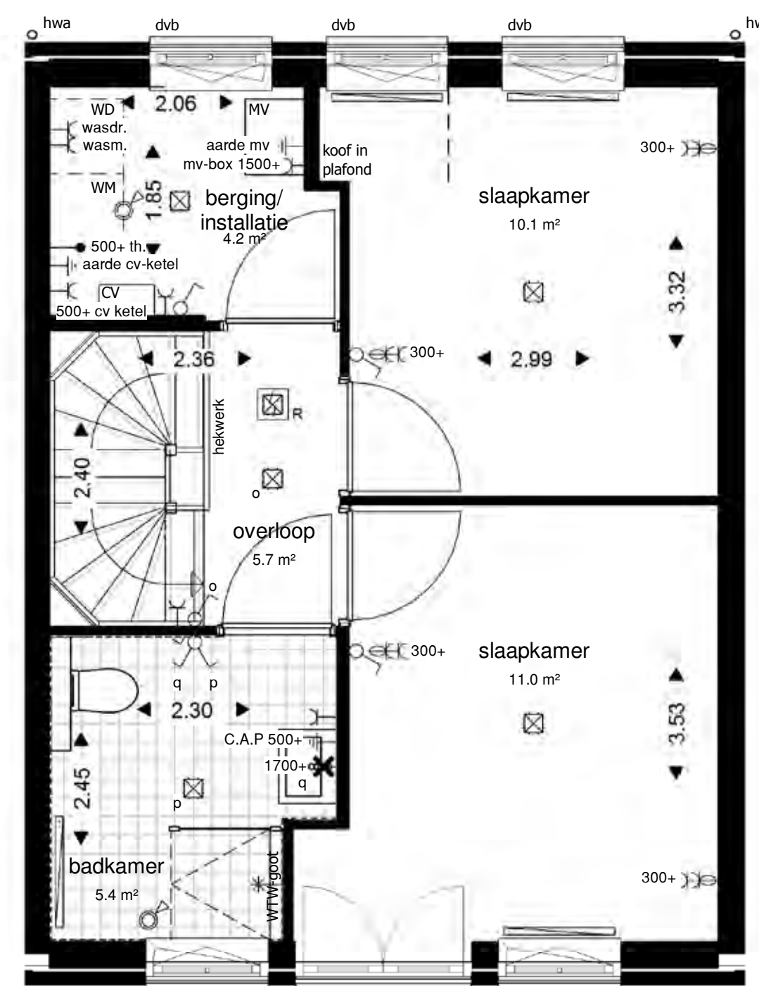
2de verdieping
