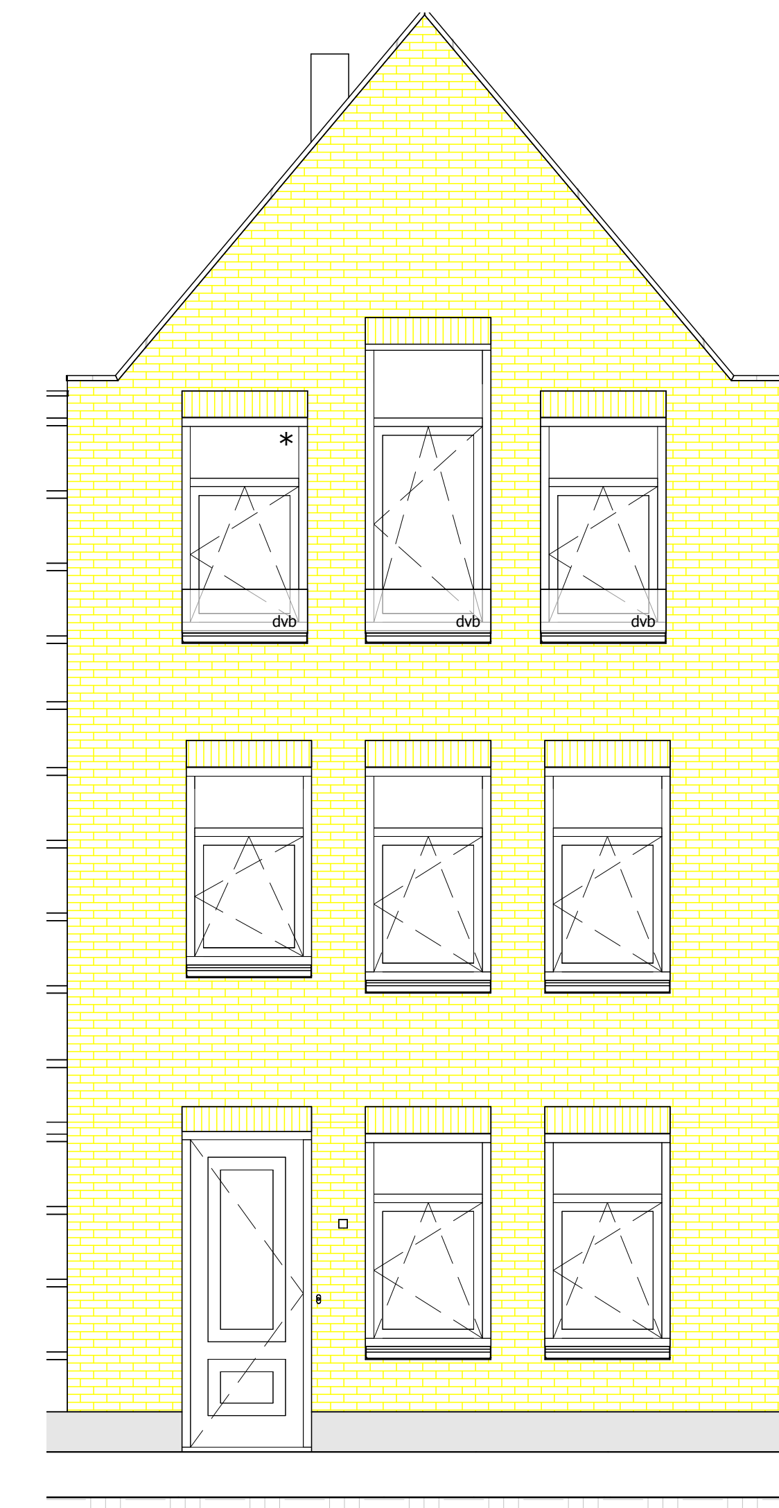
voorgevel
