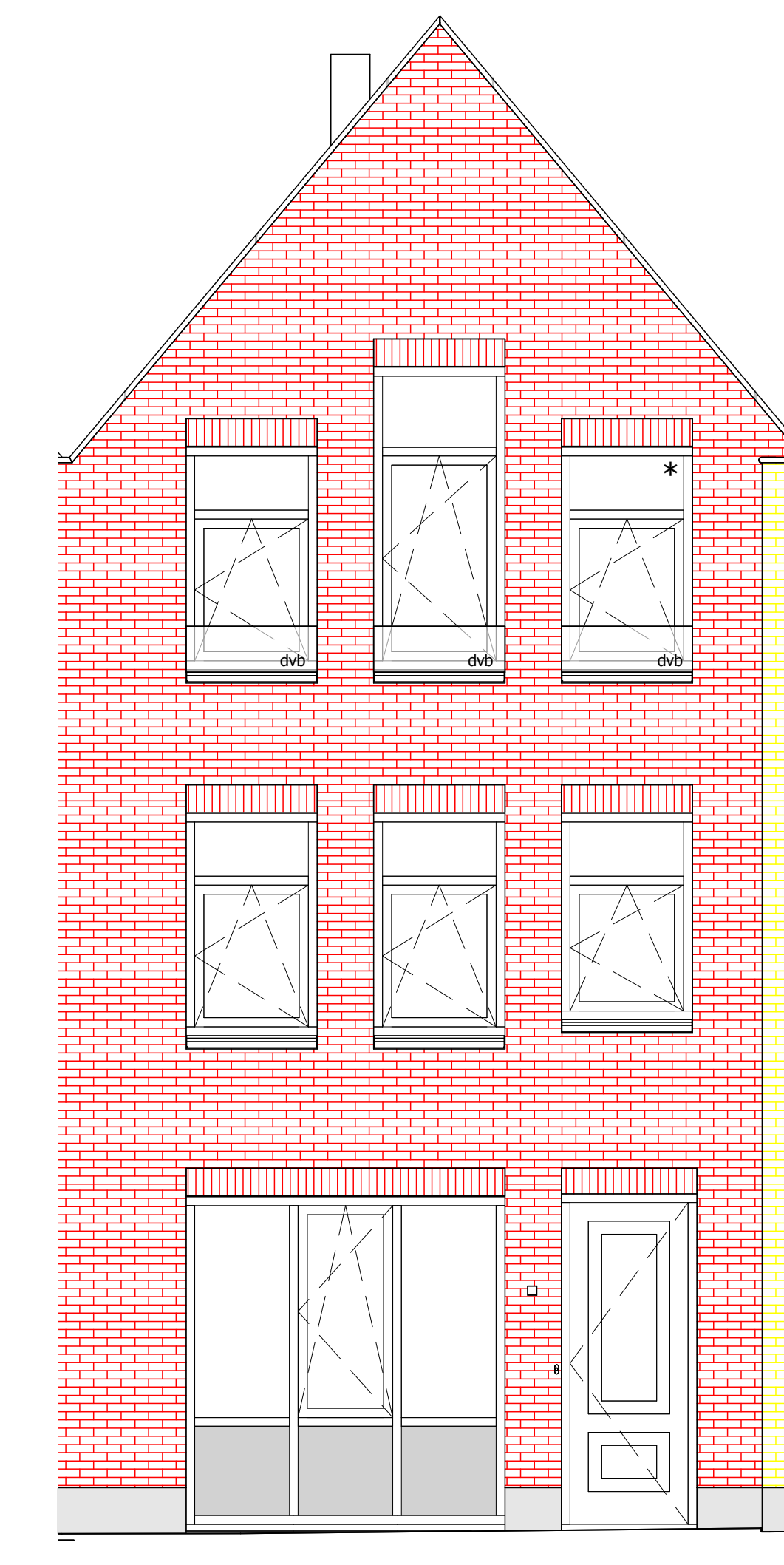
voorgevel
