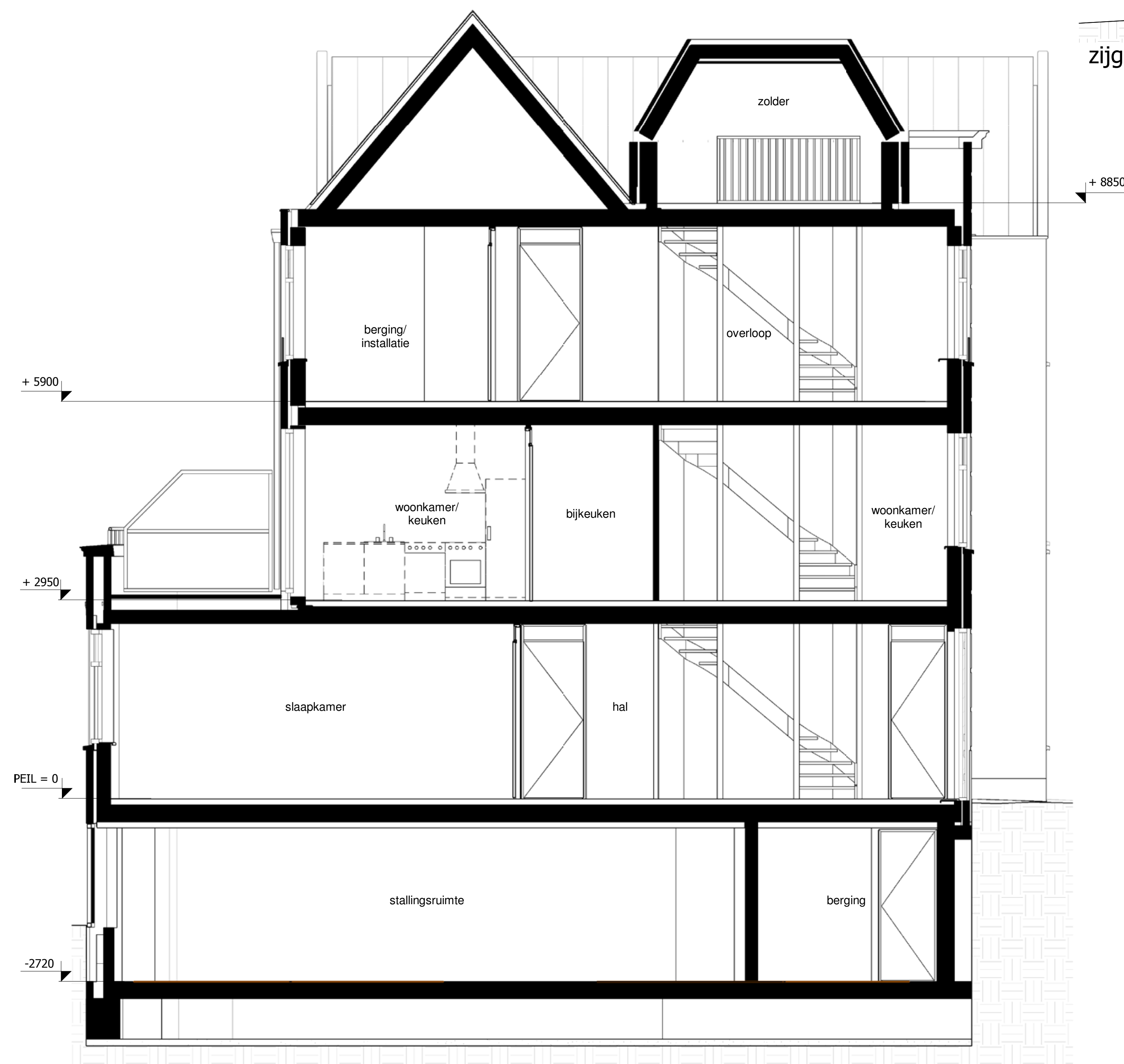
Doorsnede
