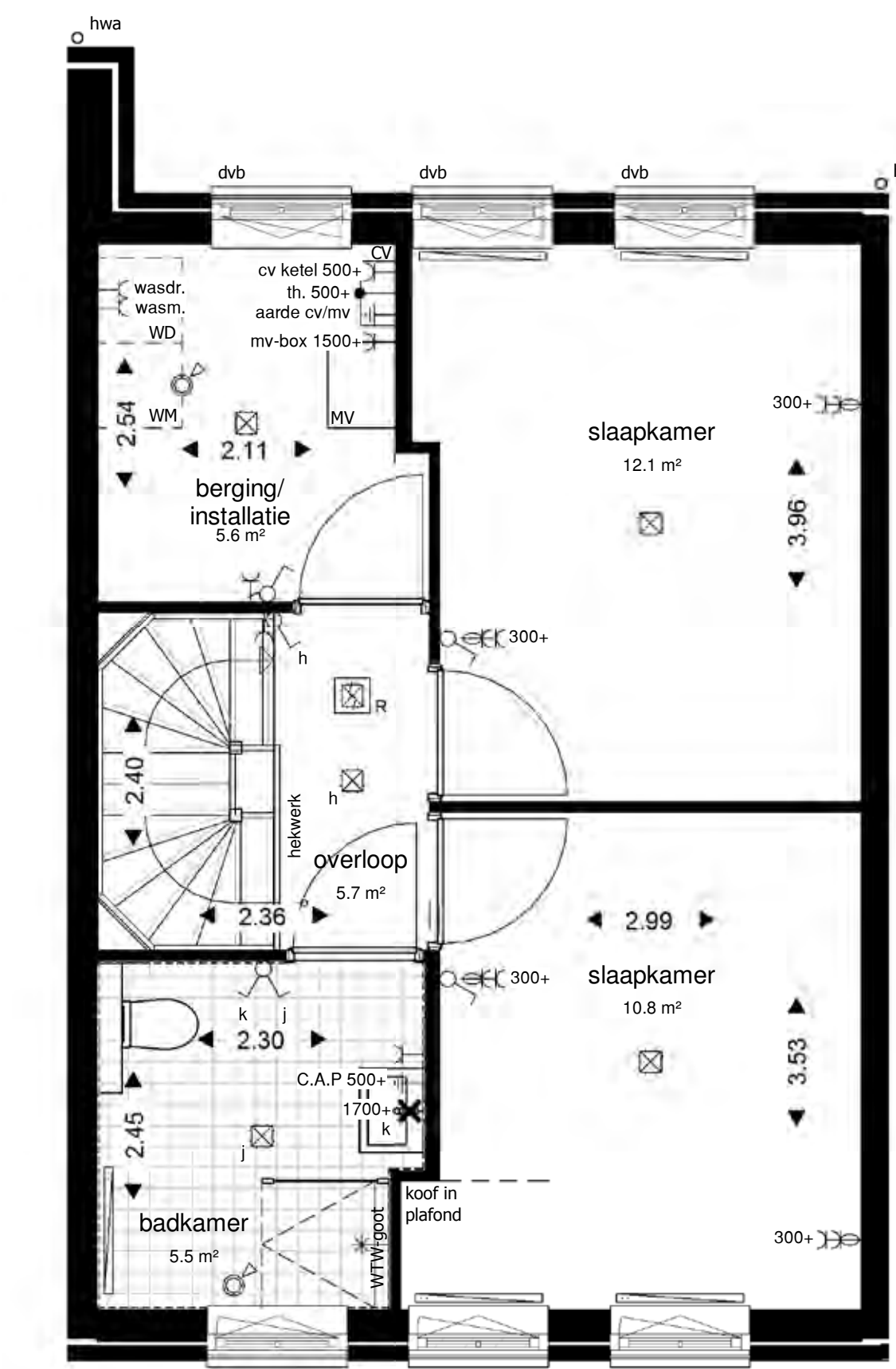
2e verdieping
