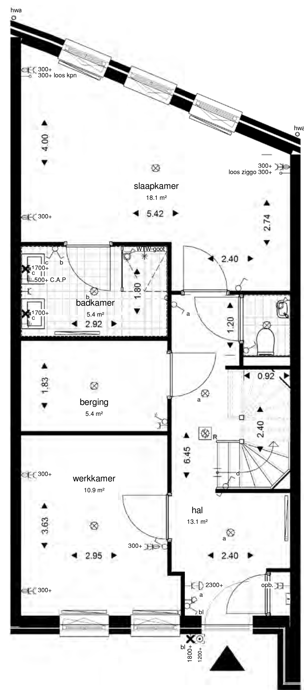
begane grond
