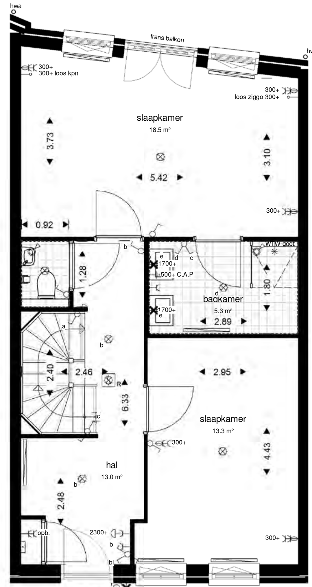
begane grond
