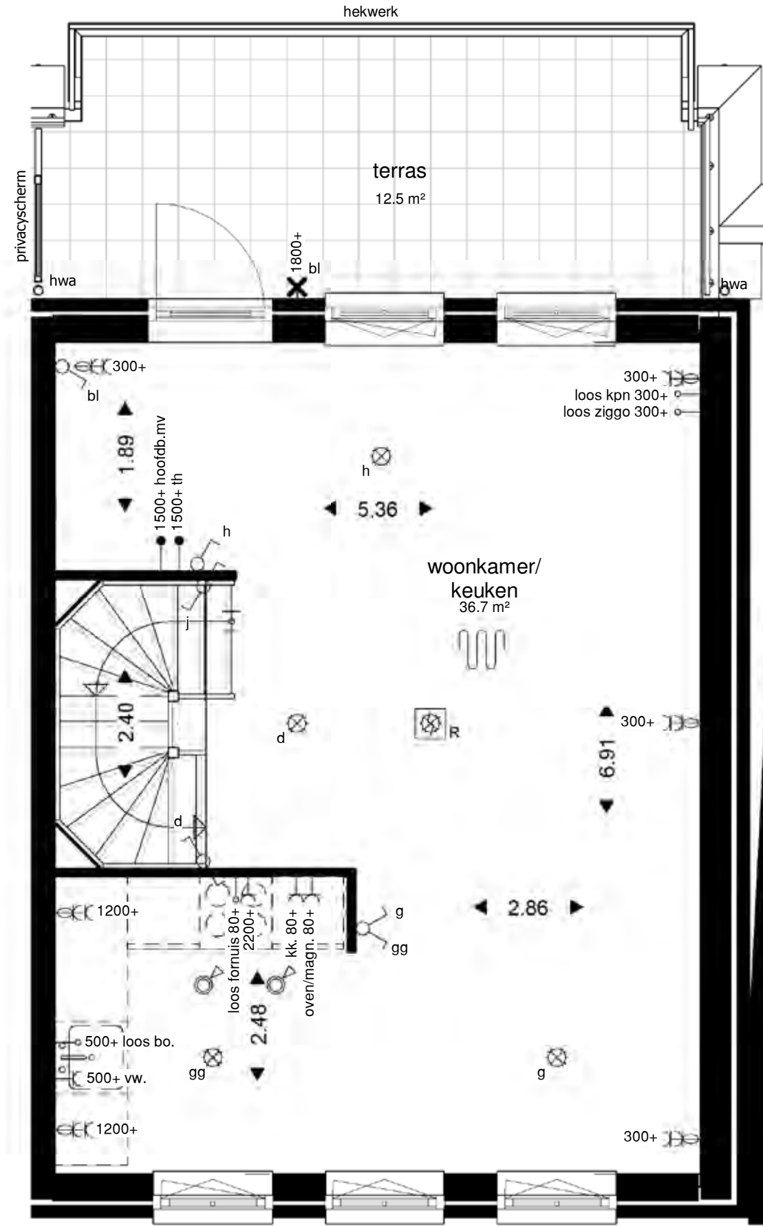
1ste verdieping
