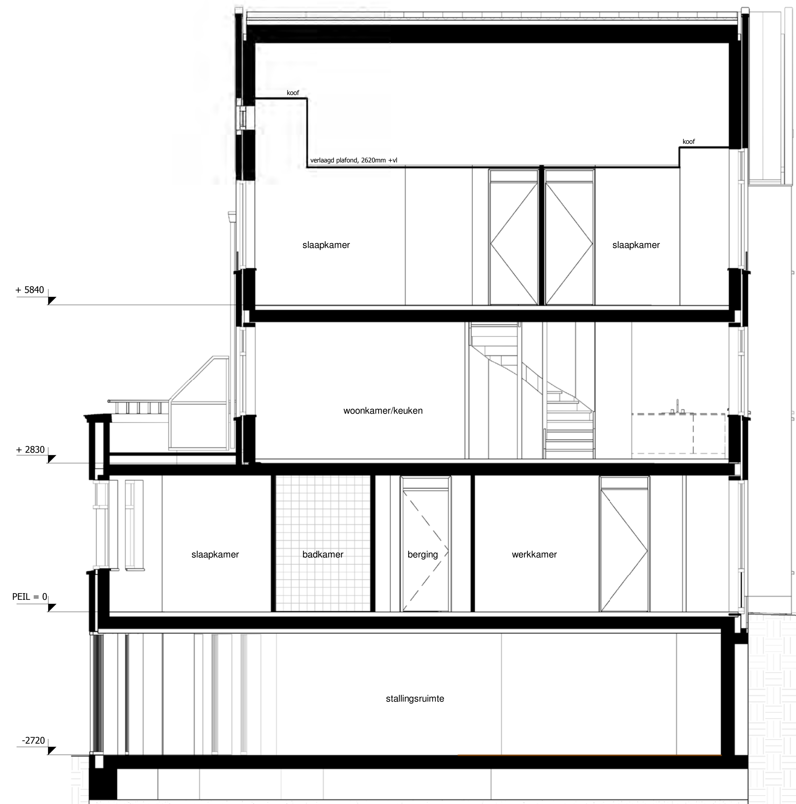
Doorsnede
