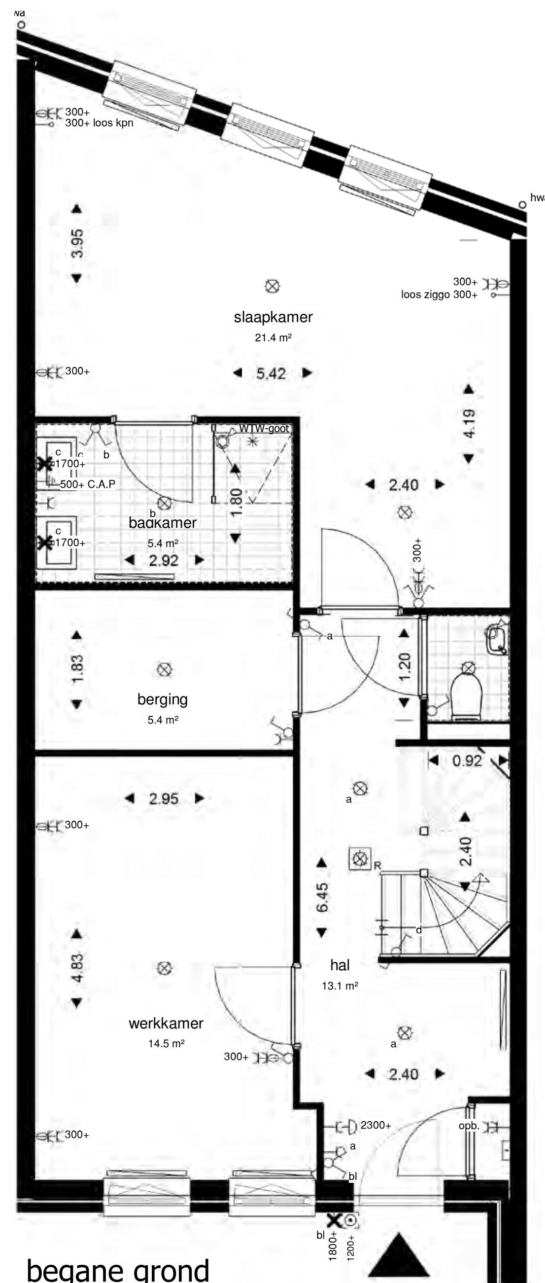
begane grond
