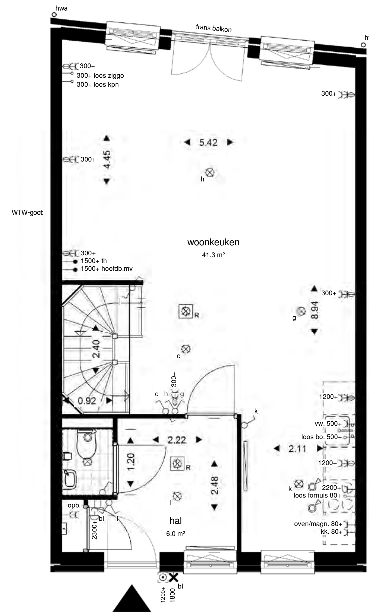
begane grond
