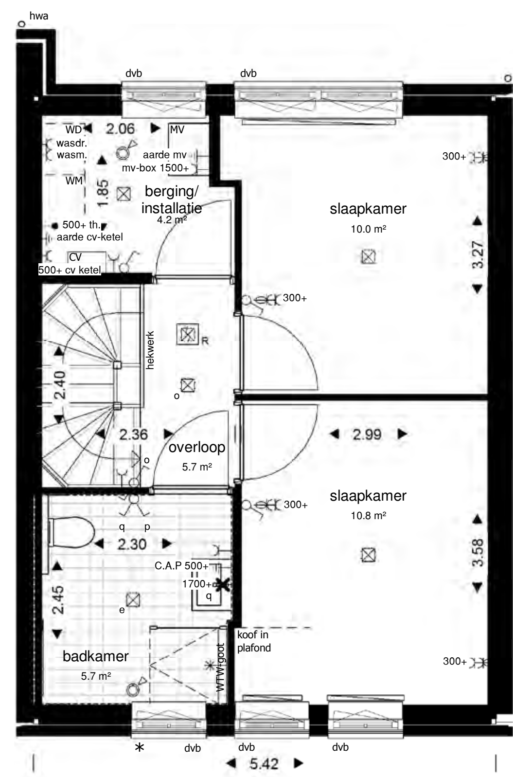
2de verdieping
