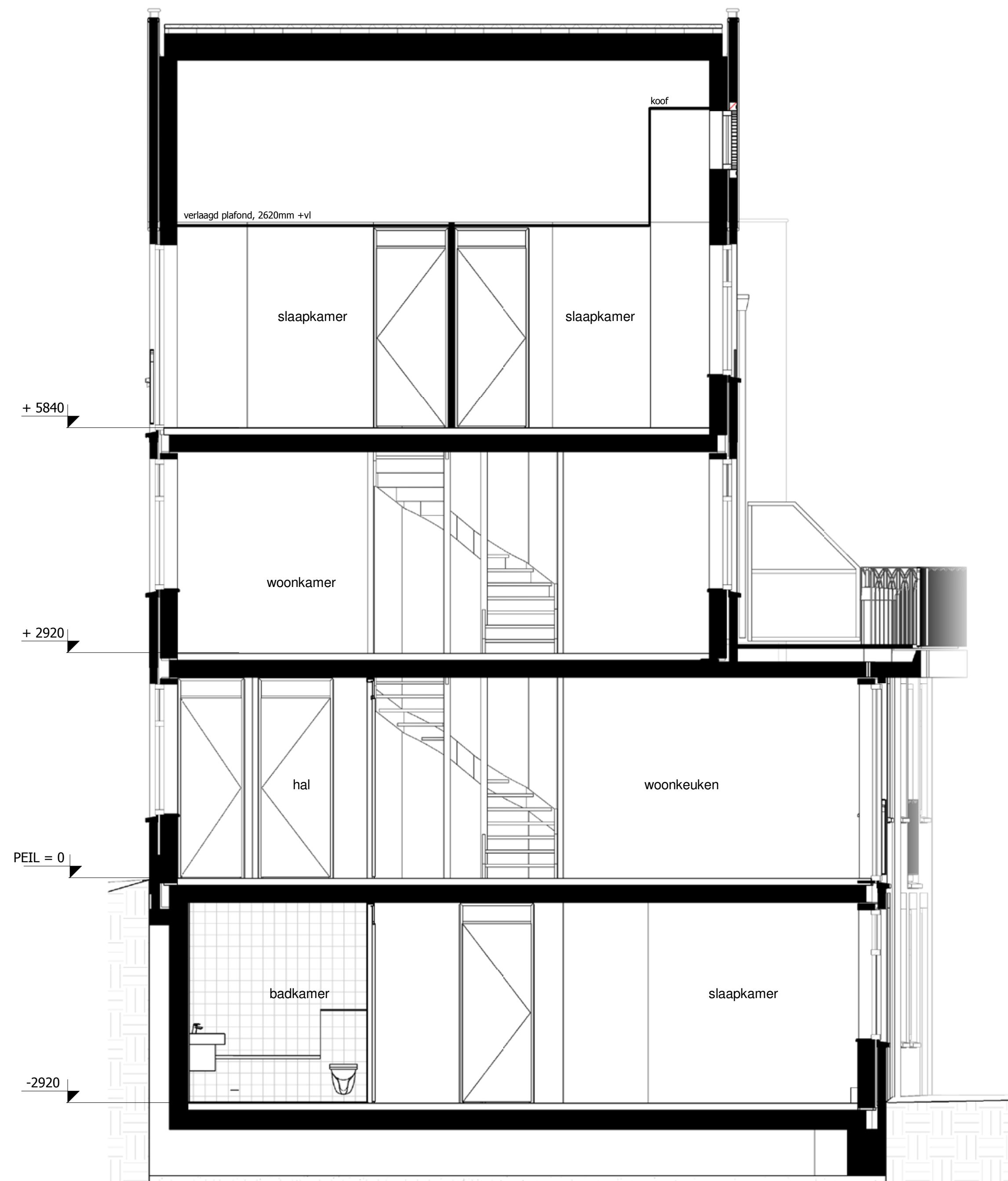
Doorsnede
