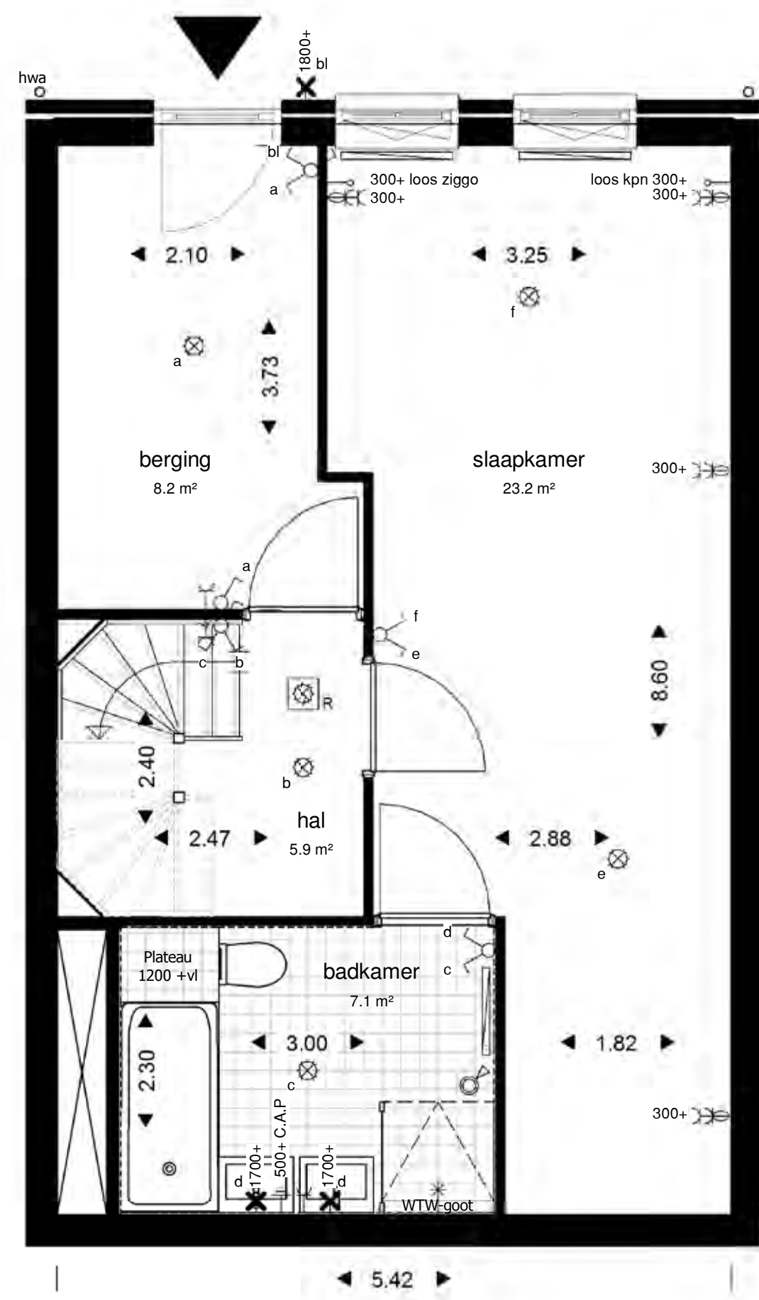
kelder
