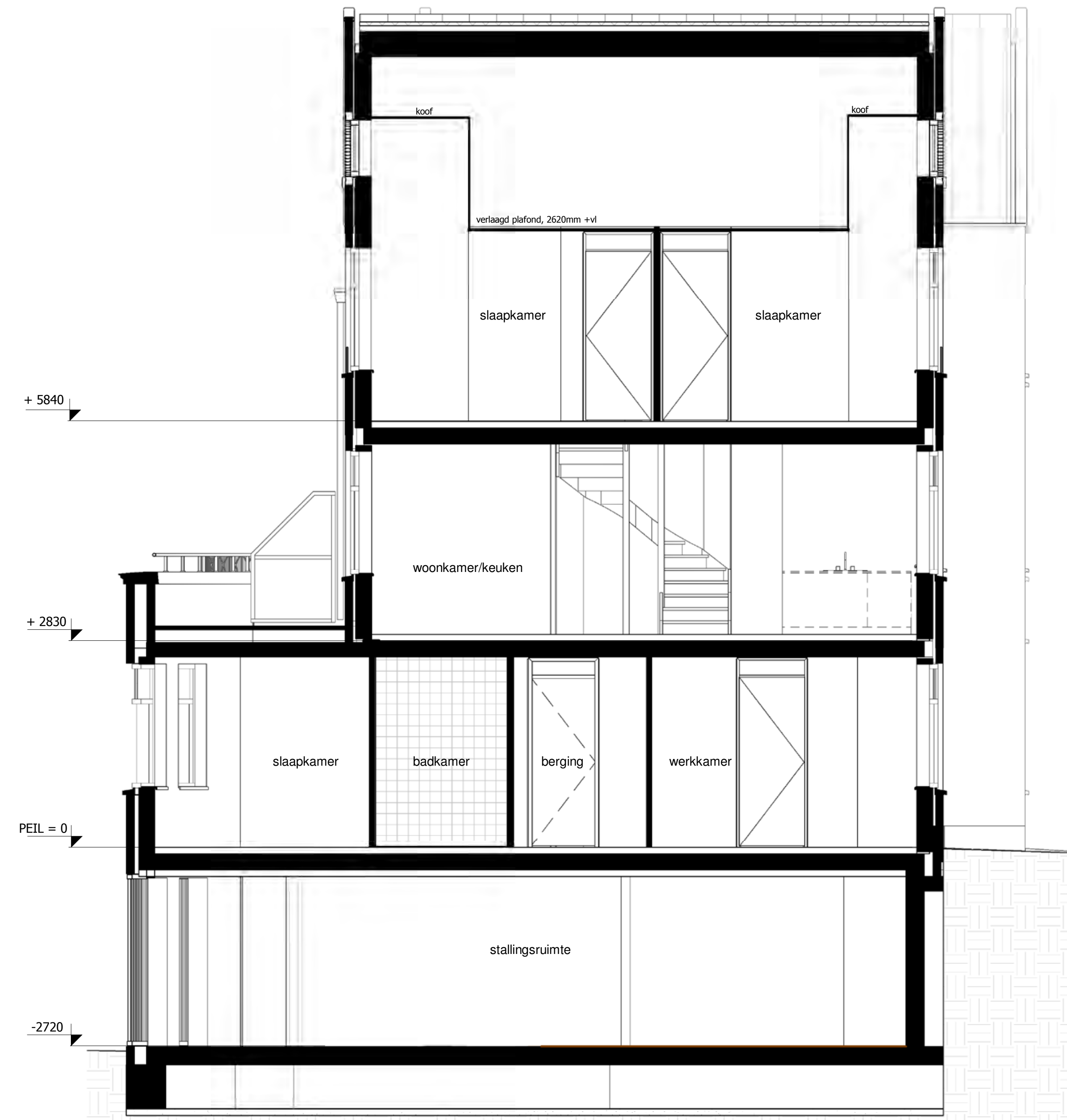
Doorsnede
