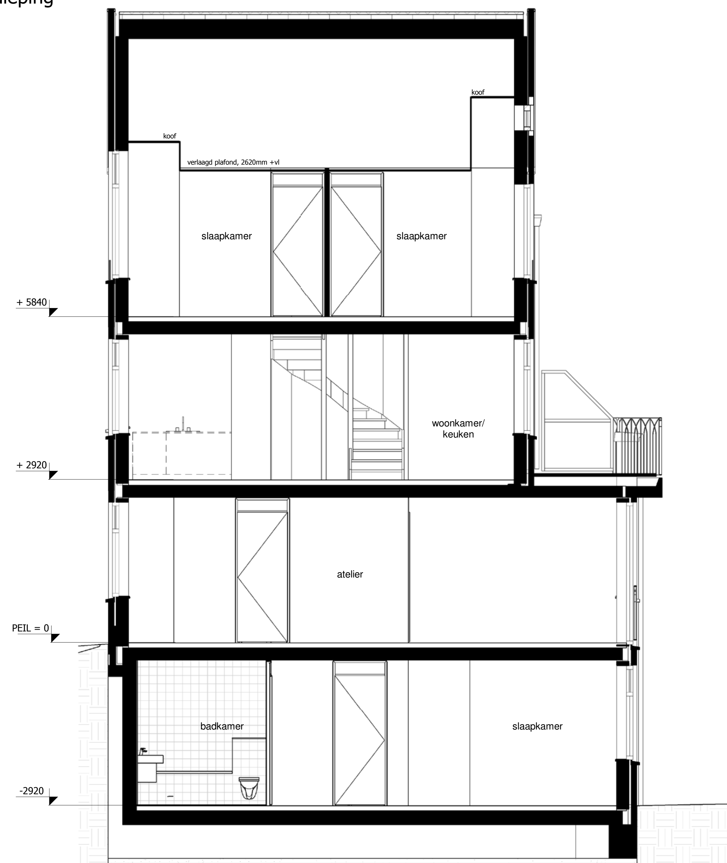
Doorsnede
