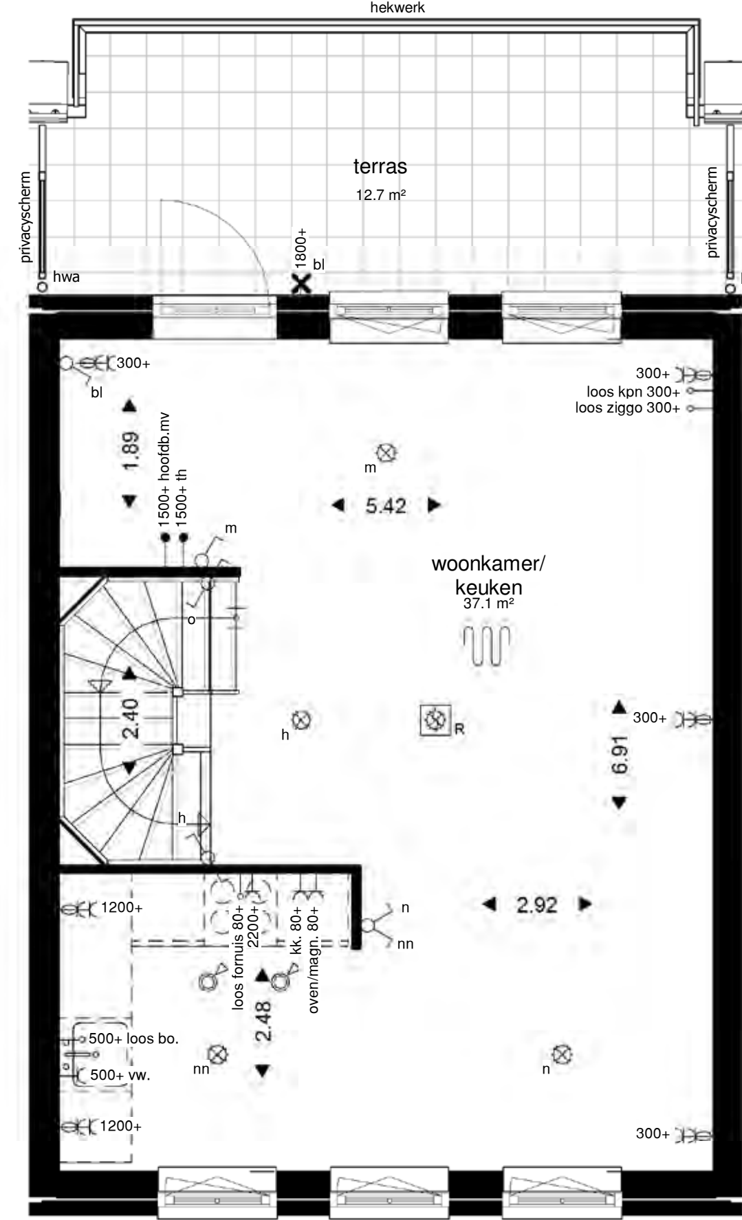
1ste verdieping
