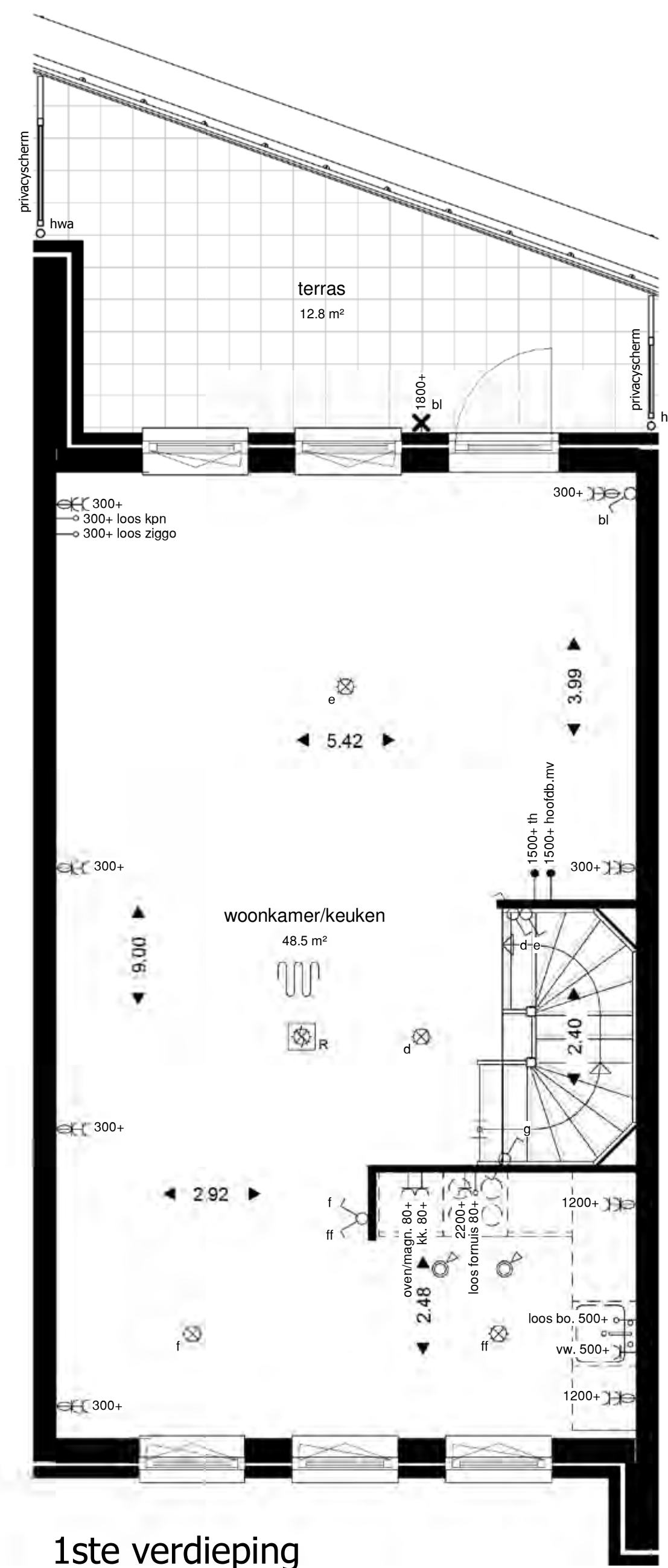
1ste verdieping
