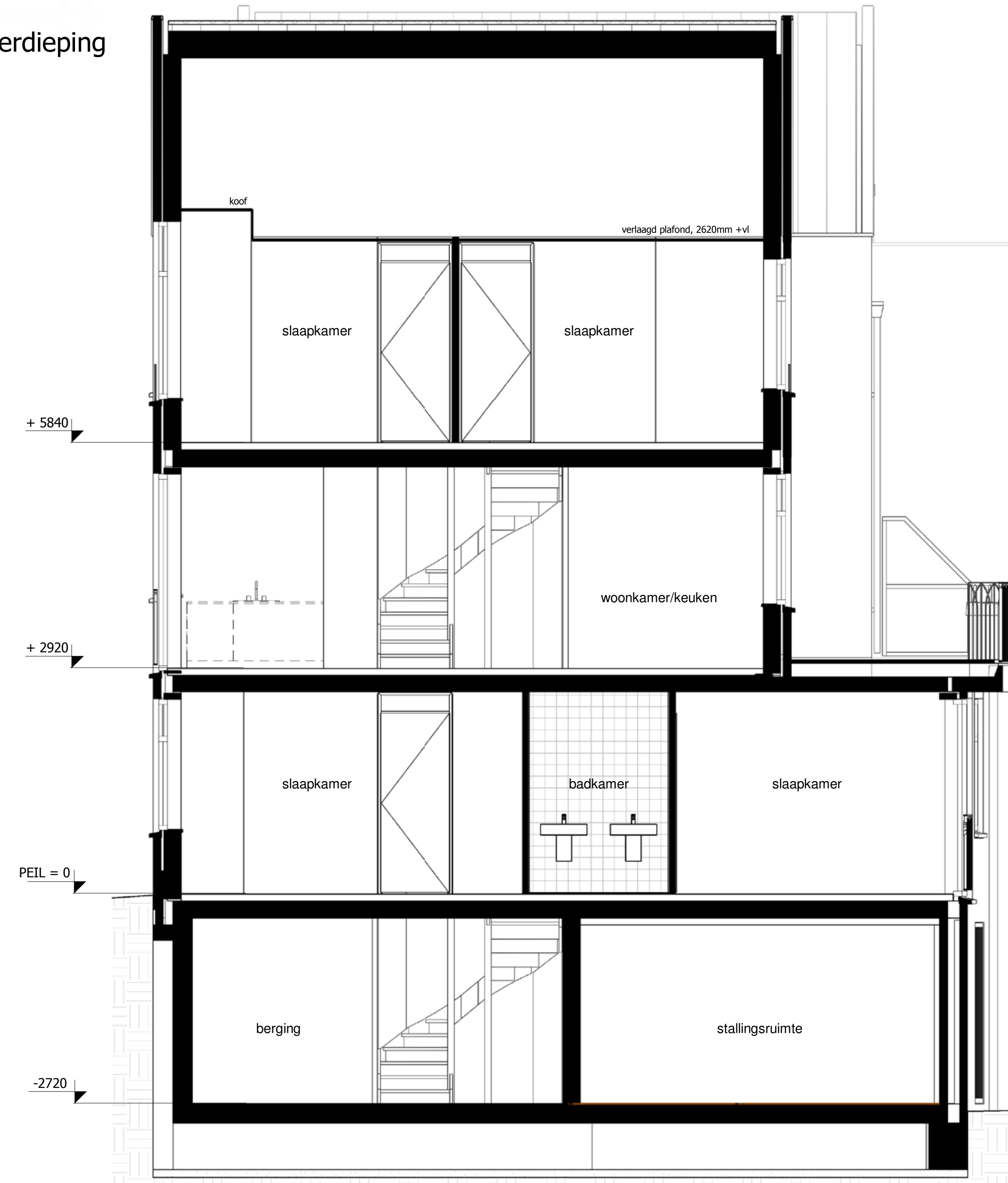
Doorsnede
