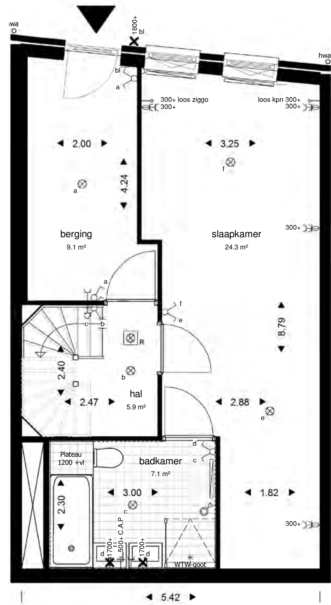
kelder
