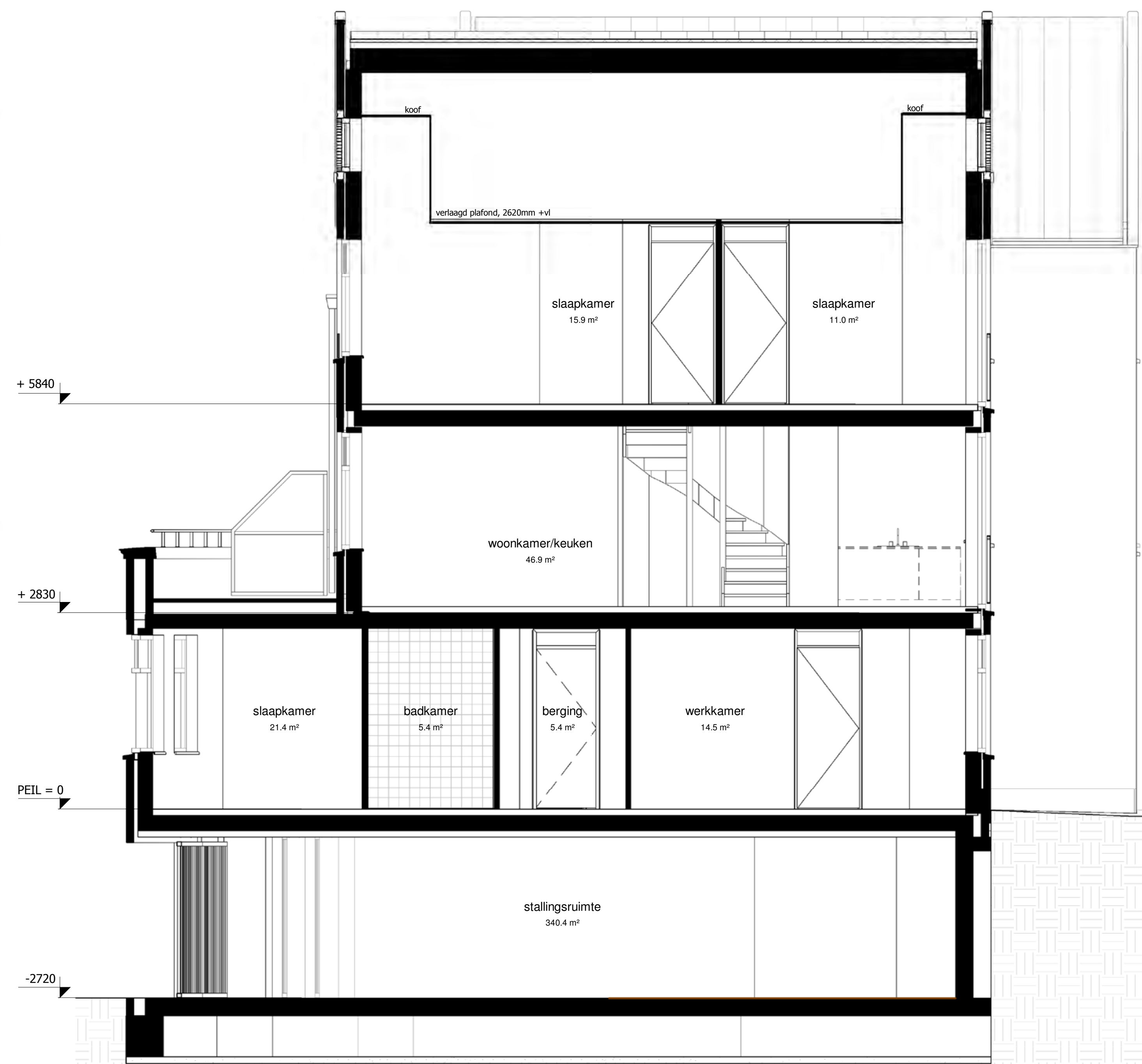
Doorsnede
