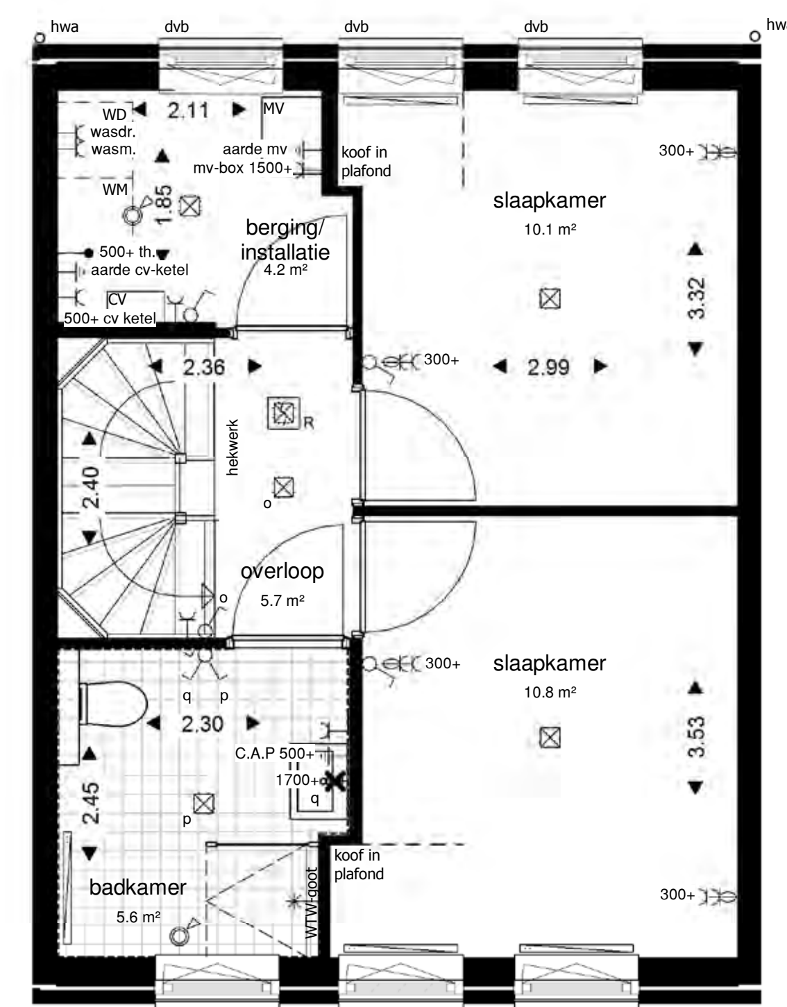
2de verdieping
