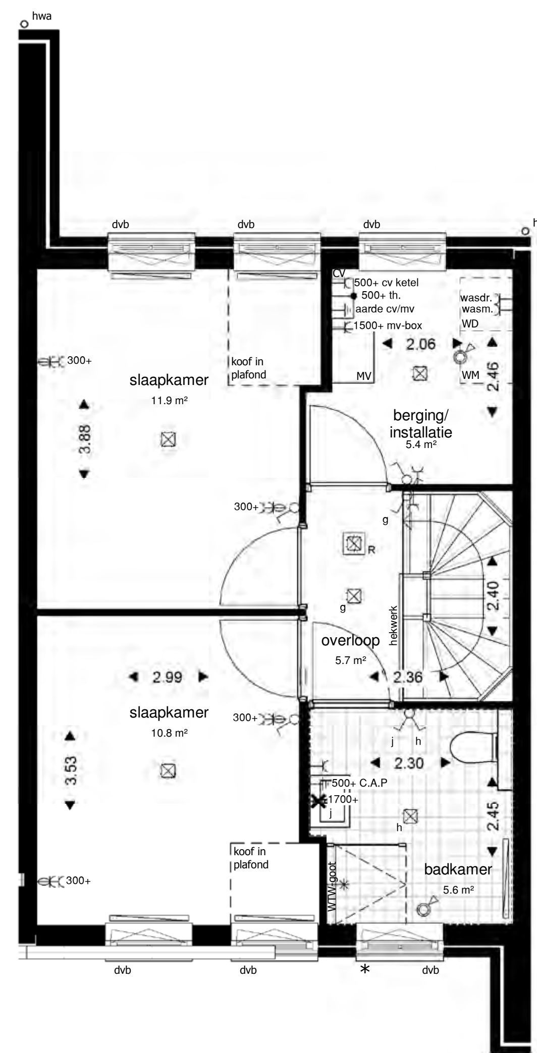
2de verdieping
