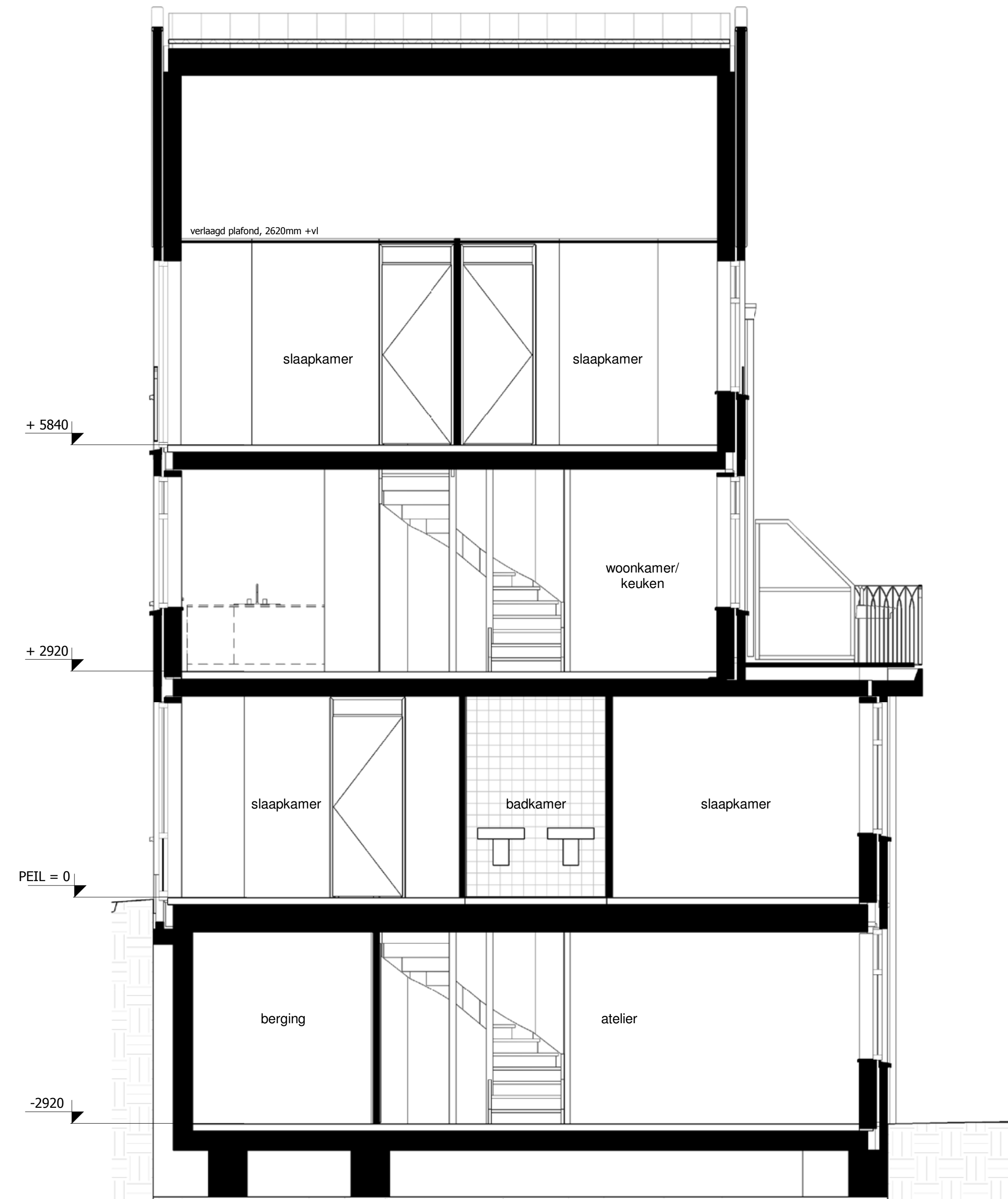
Doorsnede
