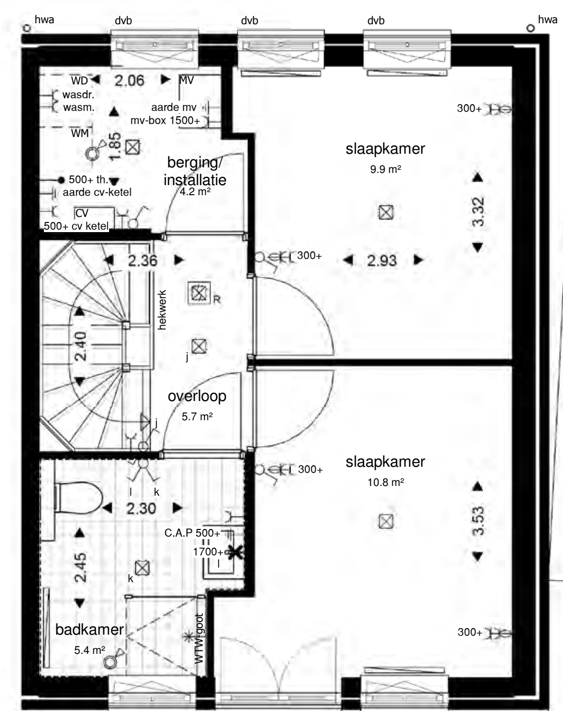
2de verdieping
