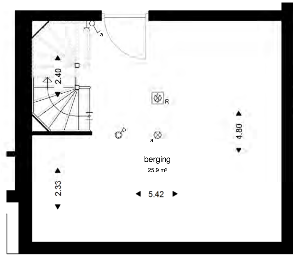
kelder
