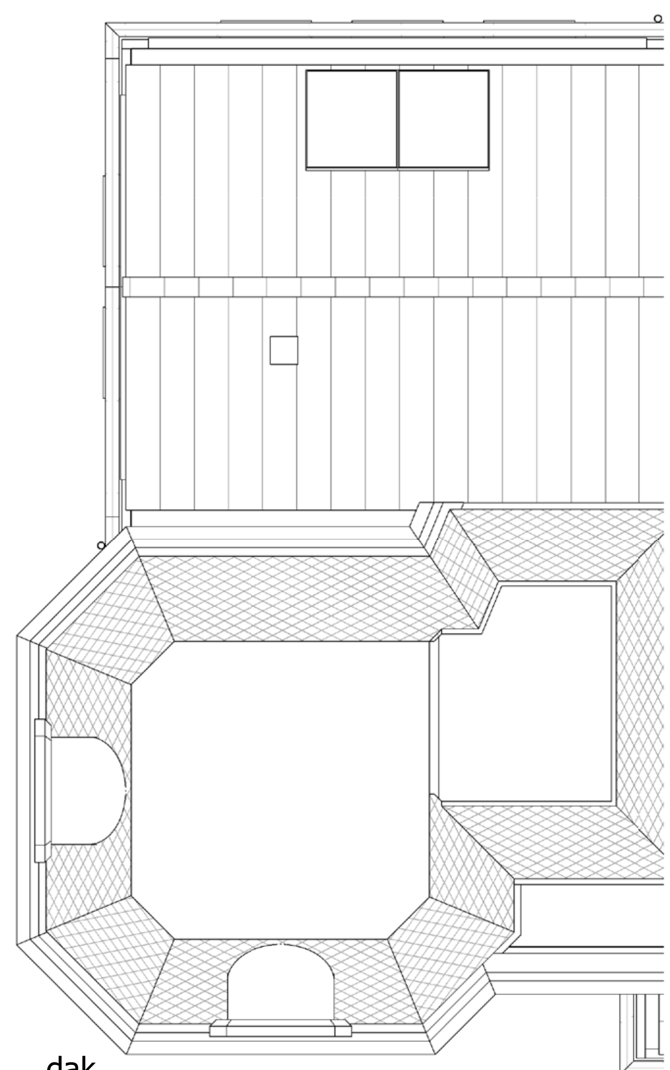
dak
