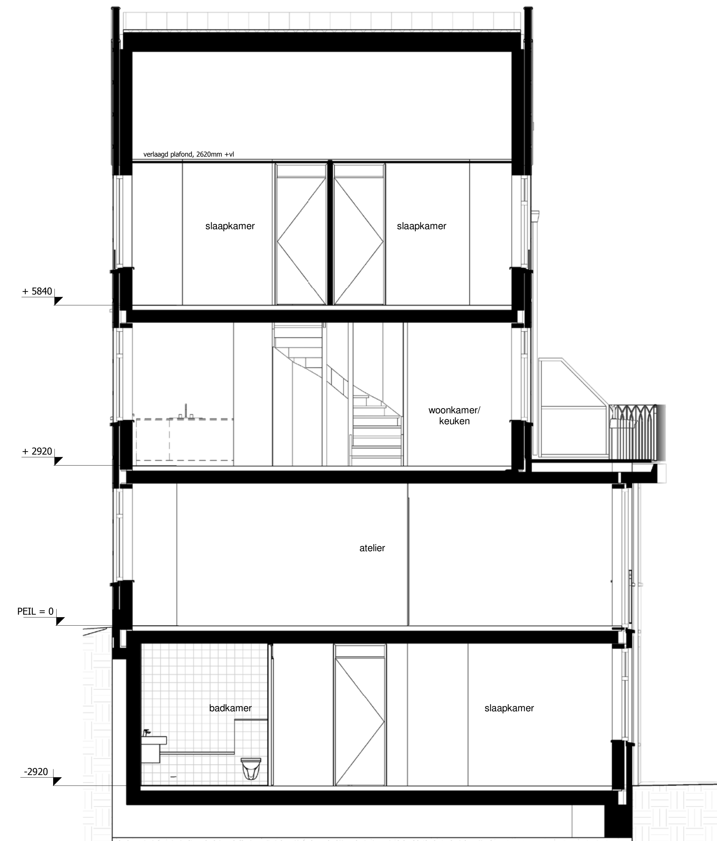
Doorsnede
