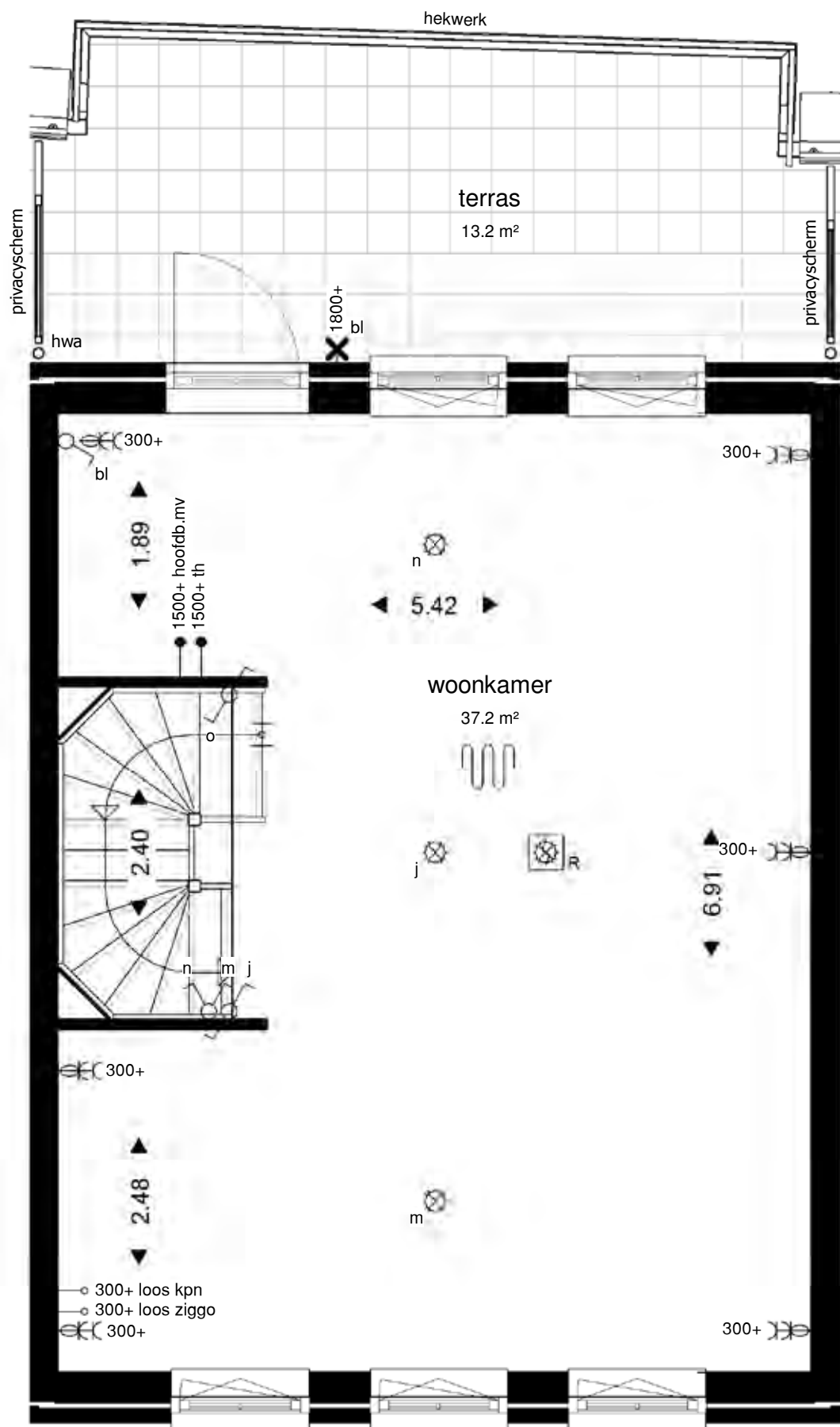
1ste verdieping
