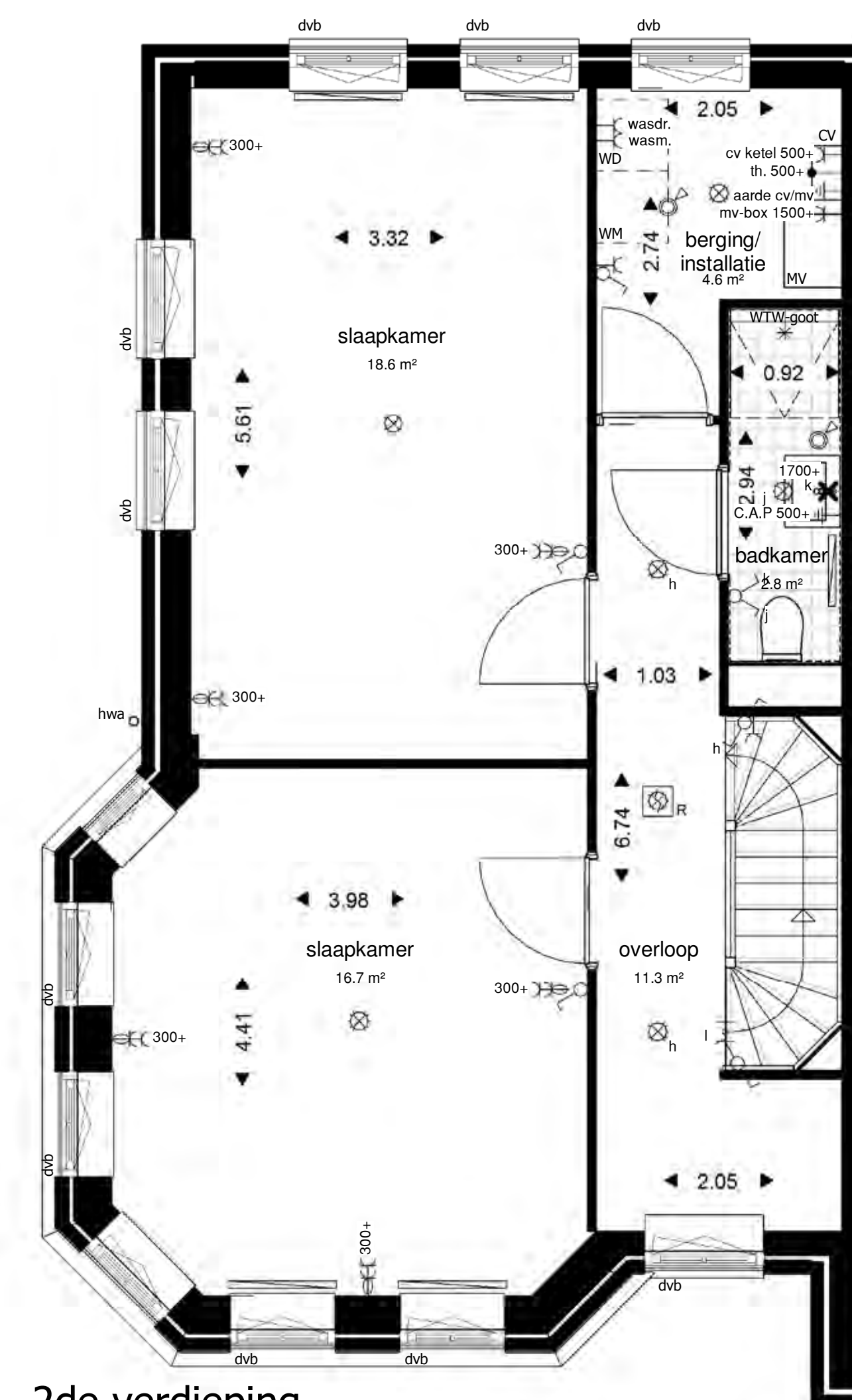
2de verdieping
