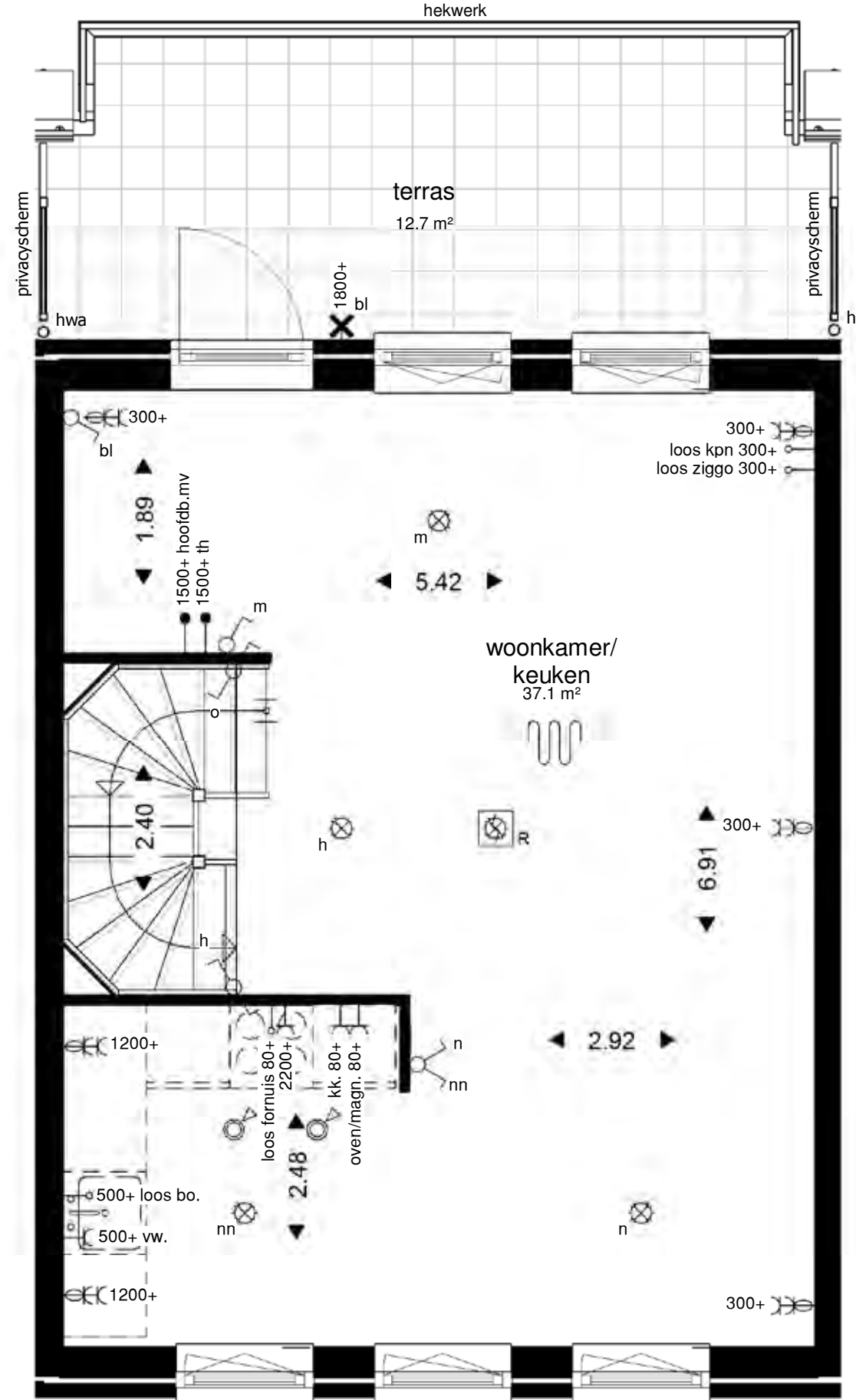
1ste verdieping
