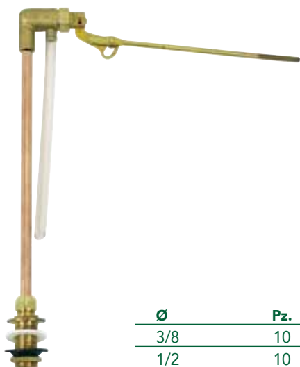
Art. 1648 Galleggiante silenzioso attacco basso
