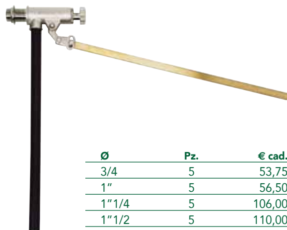
Art. 1656/A Galleggiante per alte pressione asta ottone sede inox
