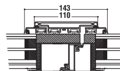
NODO CENTRALE CENTRAL NODE
