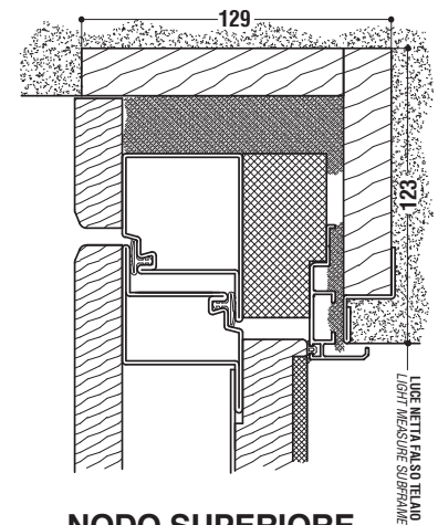
NODO SUPERIORE UPPER NODE
