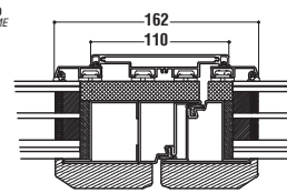
NODO CENTRALE CENTRAL NODE
