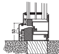
NODO INFERIORE LOWER NODE
