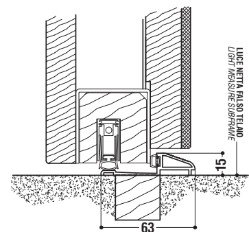
NODO INFERIORE LOWER NODE
