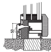
NODO INFERIORE LOWER NODE
