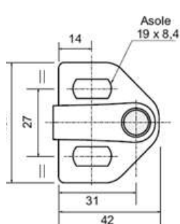
COD. 138291 PIASTRINA SPESSORE 2mm
