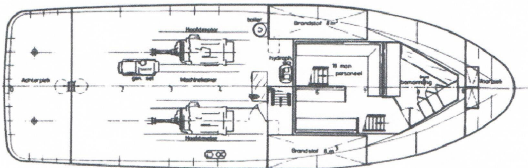
Indeling Onderdeks
